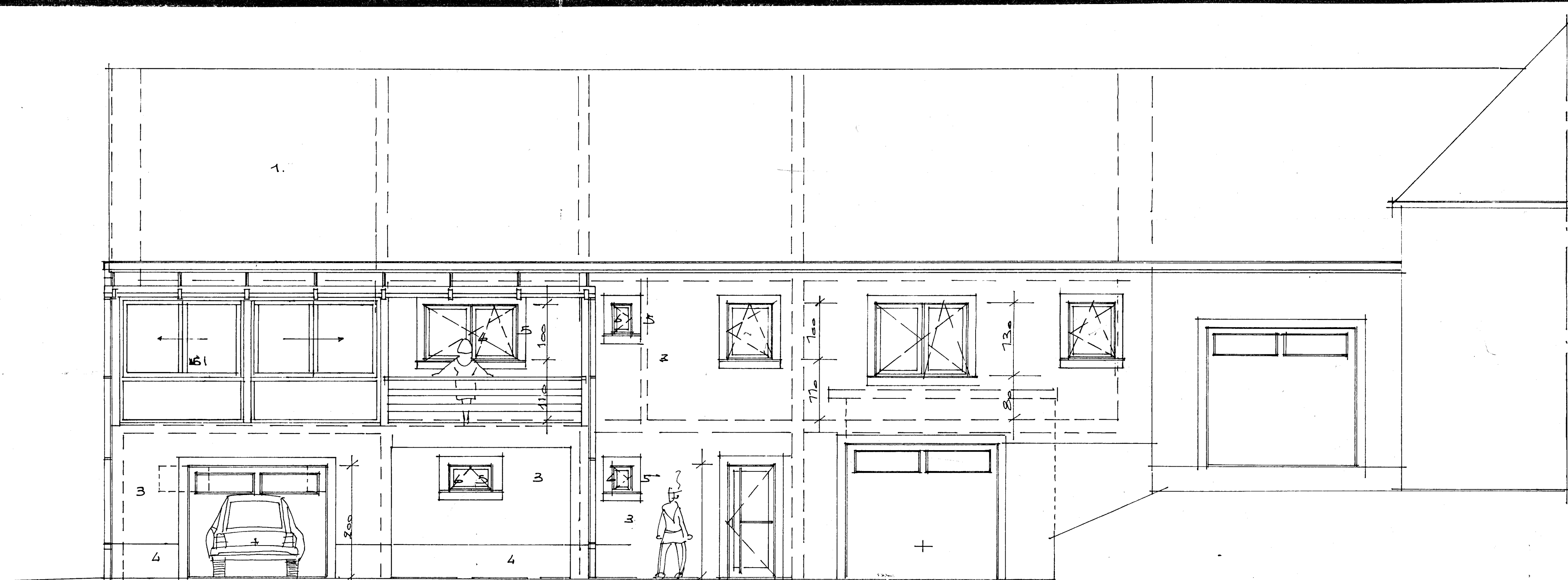
FAÇADE OUEST VERS ÉTANG
