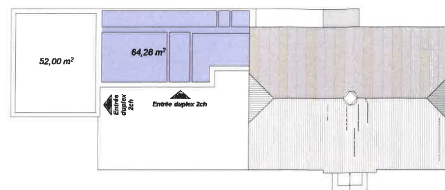
Plan de principe du rez-de-chaussée: 2*1ch / 2* 2ch / 2*rez de duplex
