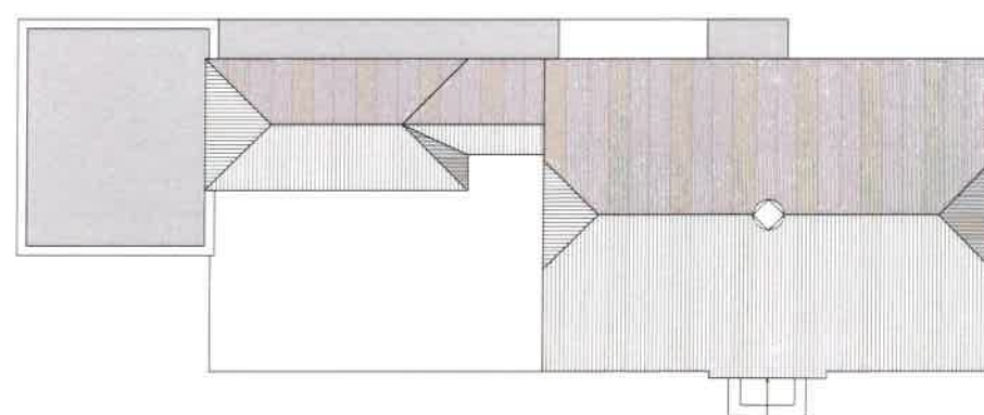
Plan de principe du rez +2: 2*1ch / 2* 2ch
