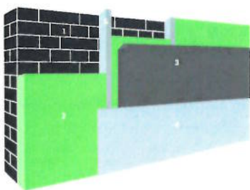
1. Buitenmuur | 2. Isolatie | 3. Vochtschermbekleding | 4. Afwerkingslaag | 5. Stijl- en regelwerk (optioneel)
