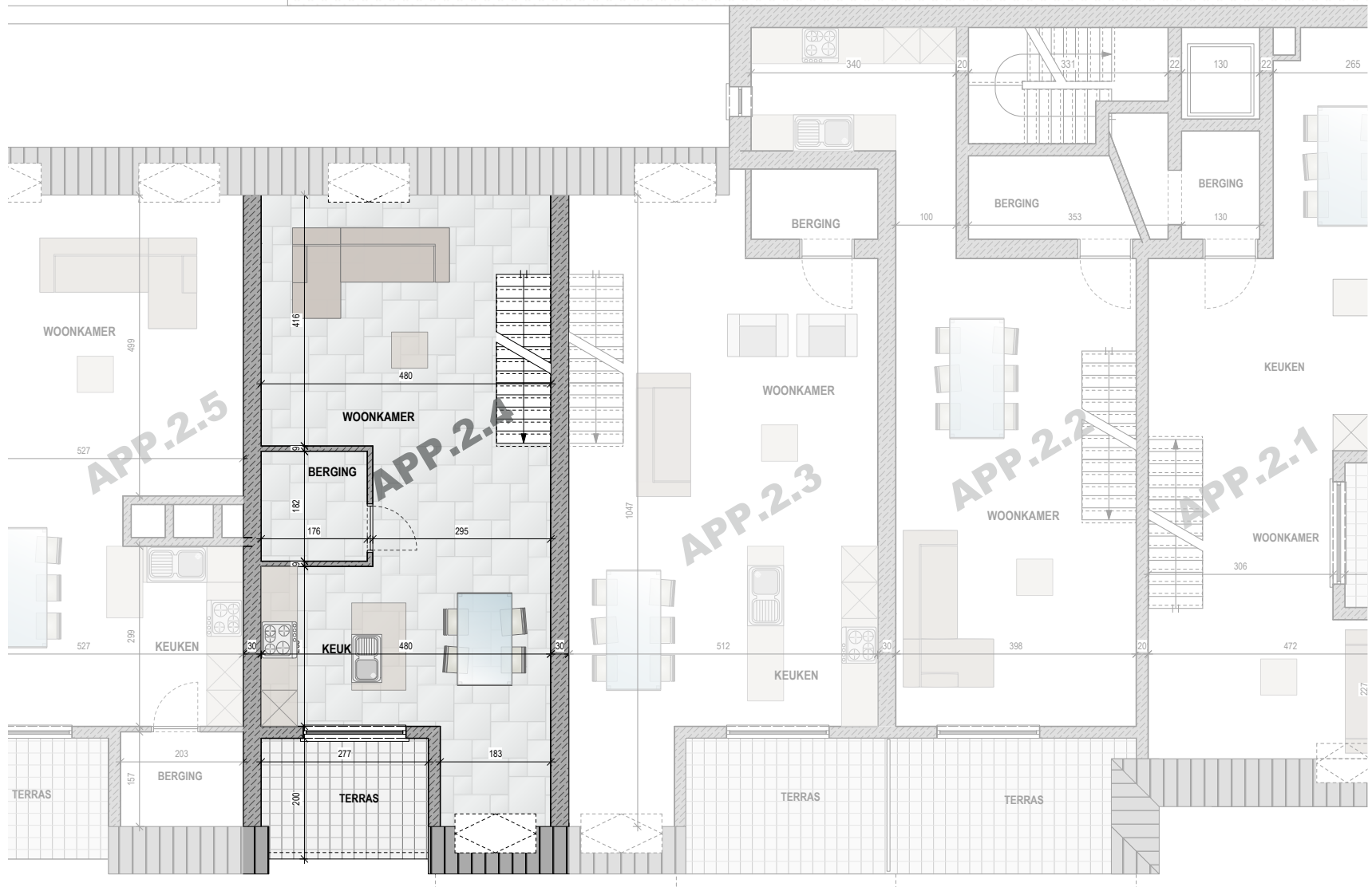
APPARTEMENT 2.1 RESIDENTIE DE POST GRONDPLAN NIVEAU 3
