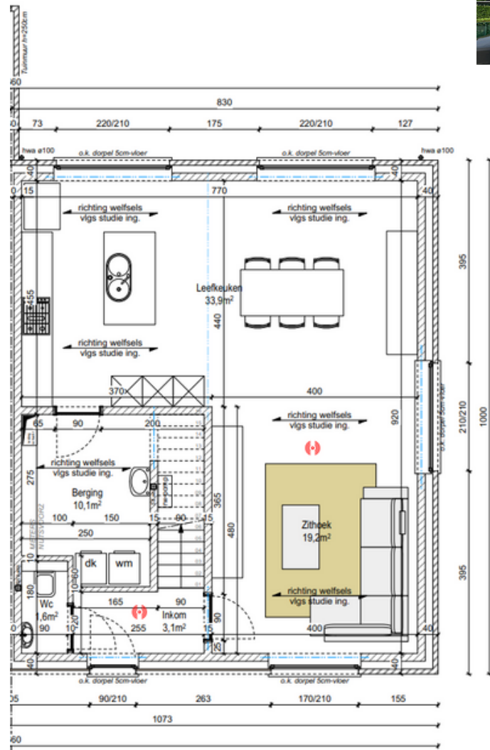
GELIJKVLOERS
