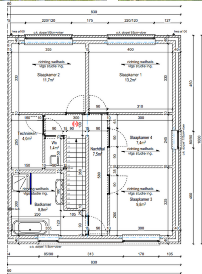
EERSTE VERDIEPING
