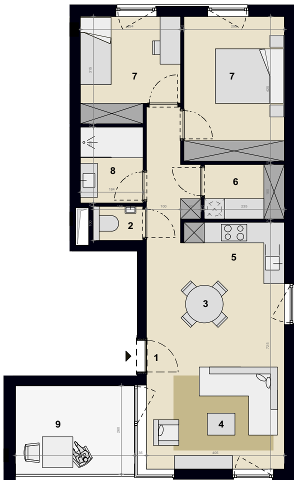
GRONDPLAN
