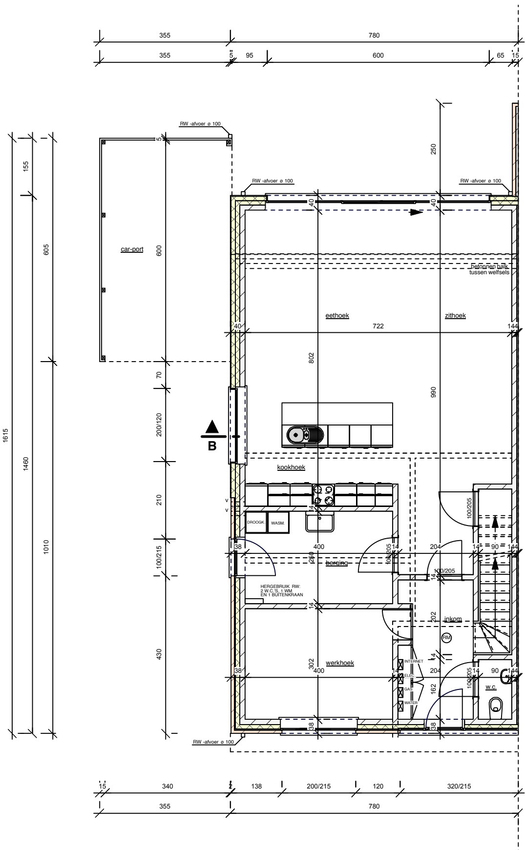
GRONDPLAN (schaal 1/100)
