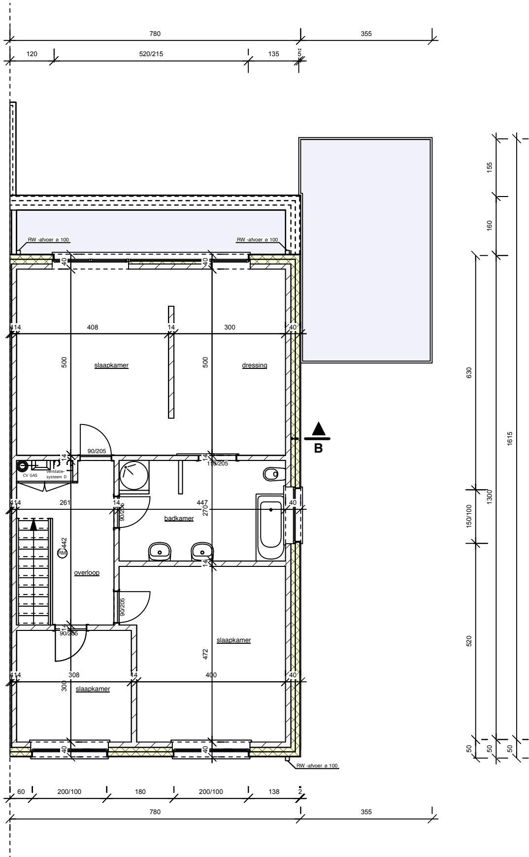
VERDIEPINGSPLAN (schaal 1/100)
