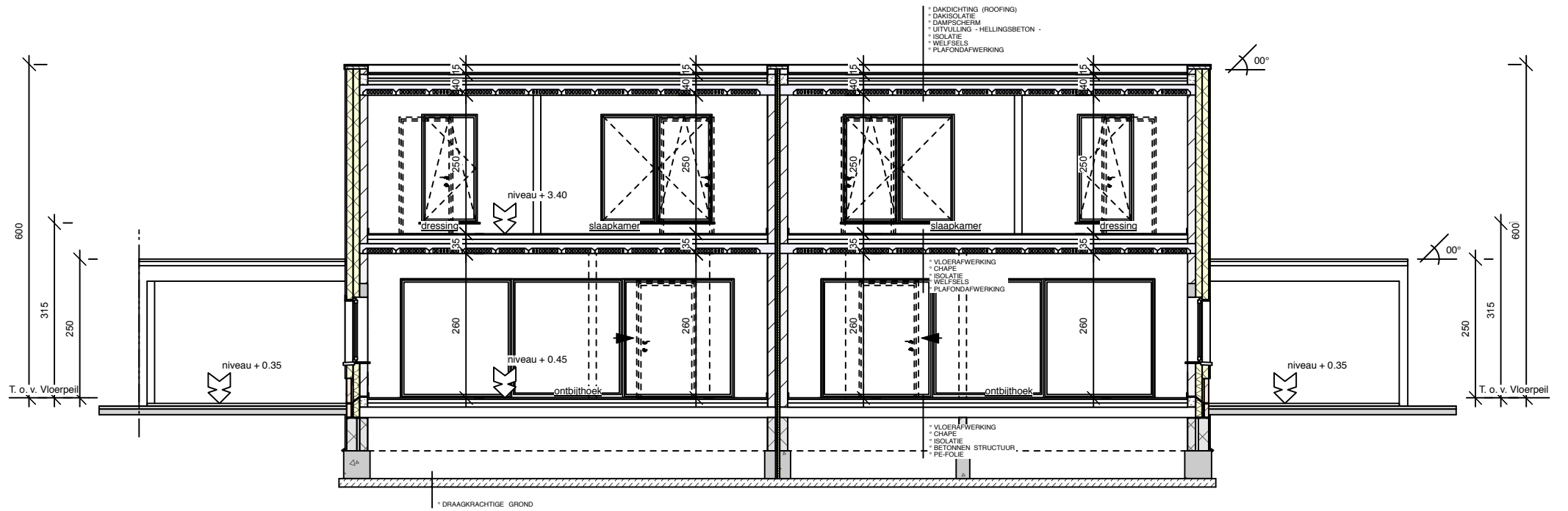
SNEDE BB (schaal 1/100)
