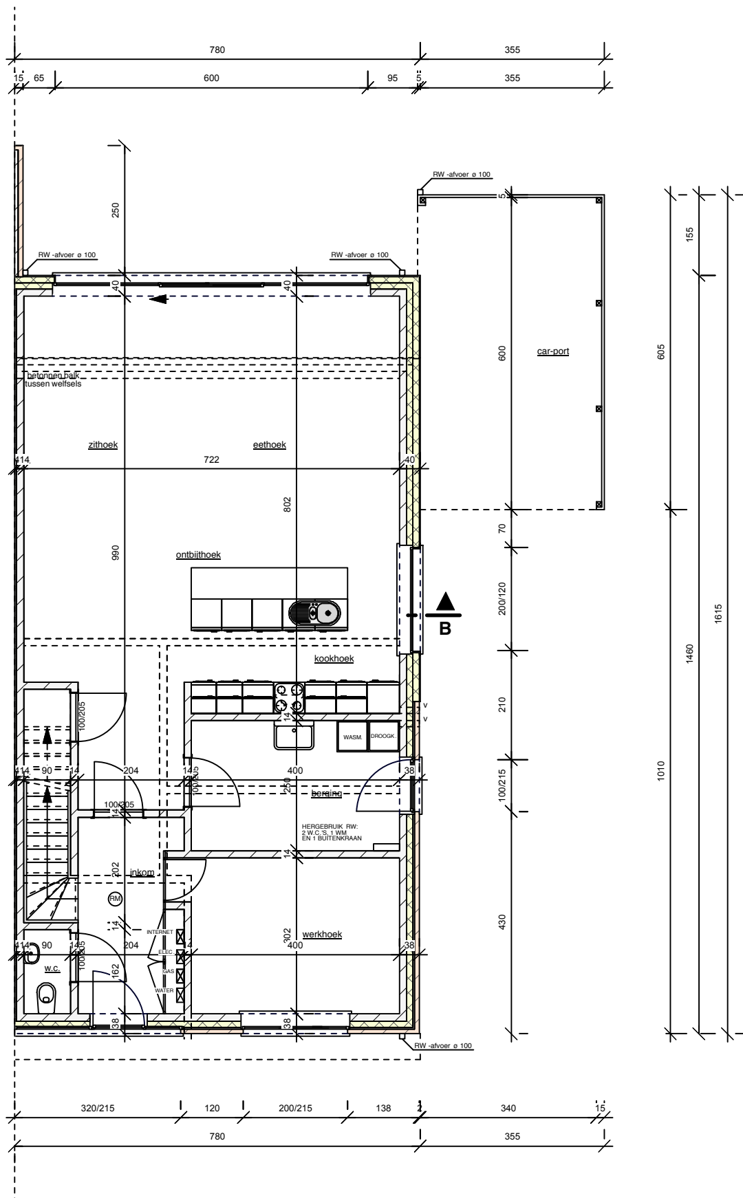
GRONDPLAN (schaal 1/100)
