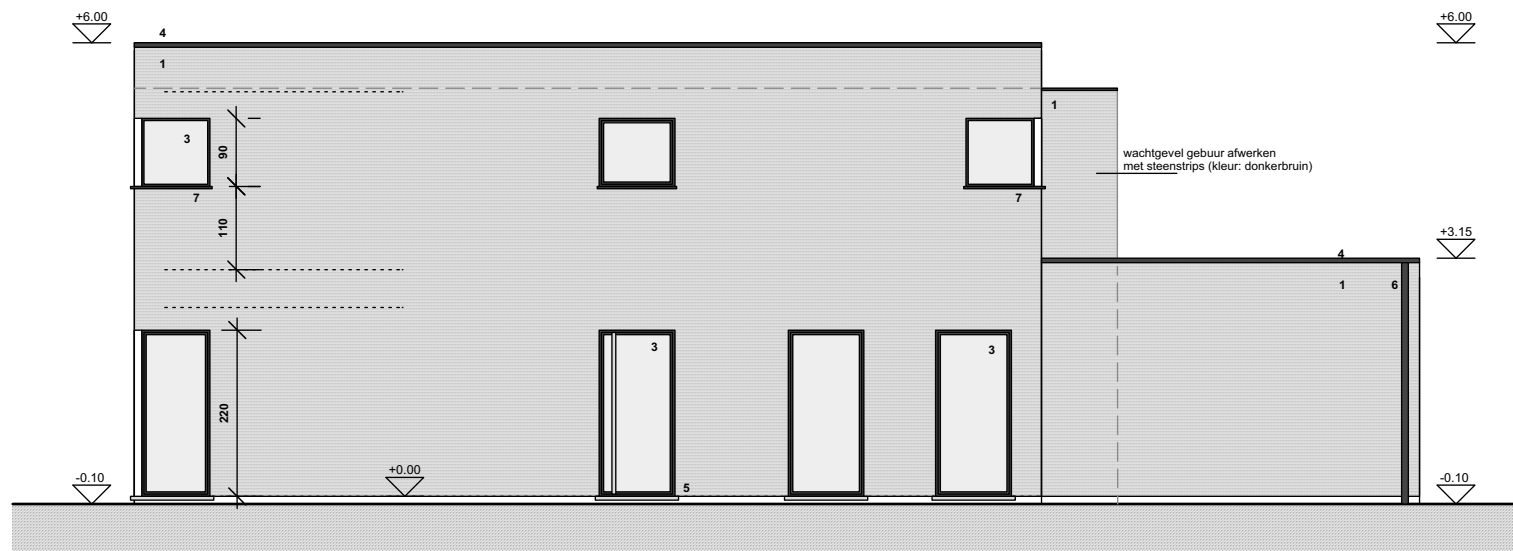
RECHTERGEVEL
