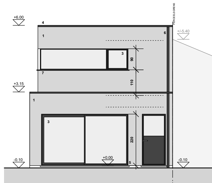
ACHTERGEVEL
