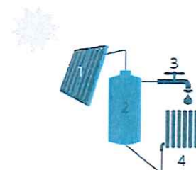
1. Zonnecollector | 2. Opslagvat zonnecollector | 3. Sanitair warm water | 4. Afgifte-element voor ruimteverwarming (optioneel)
