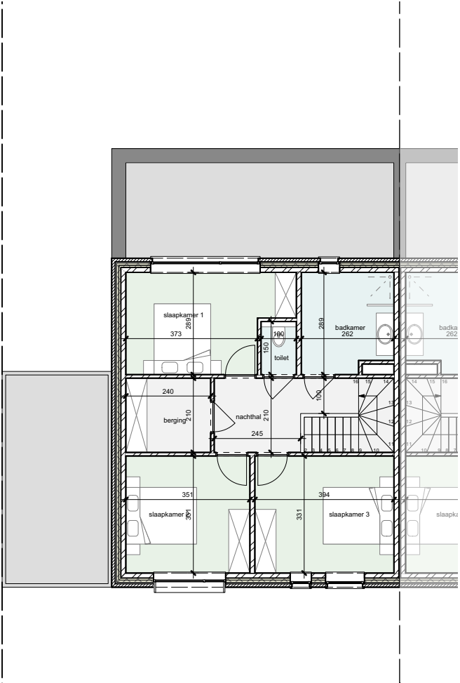
Verdieping 1
