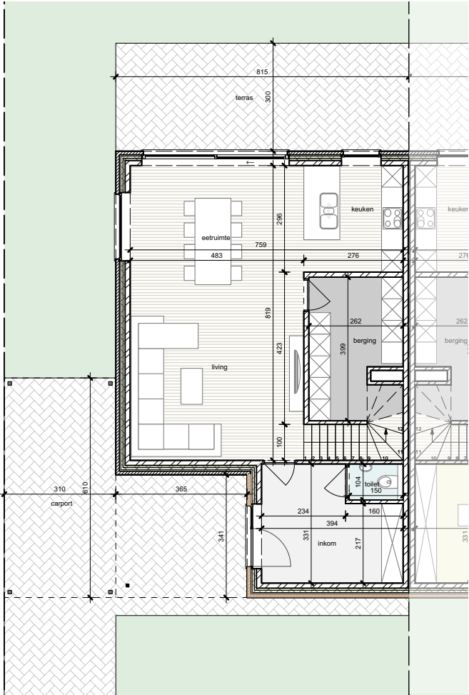
Gelijkvloers
