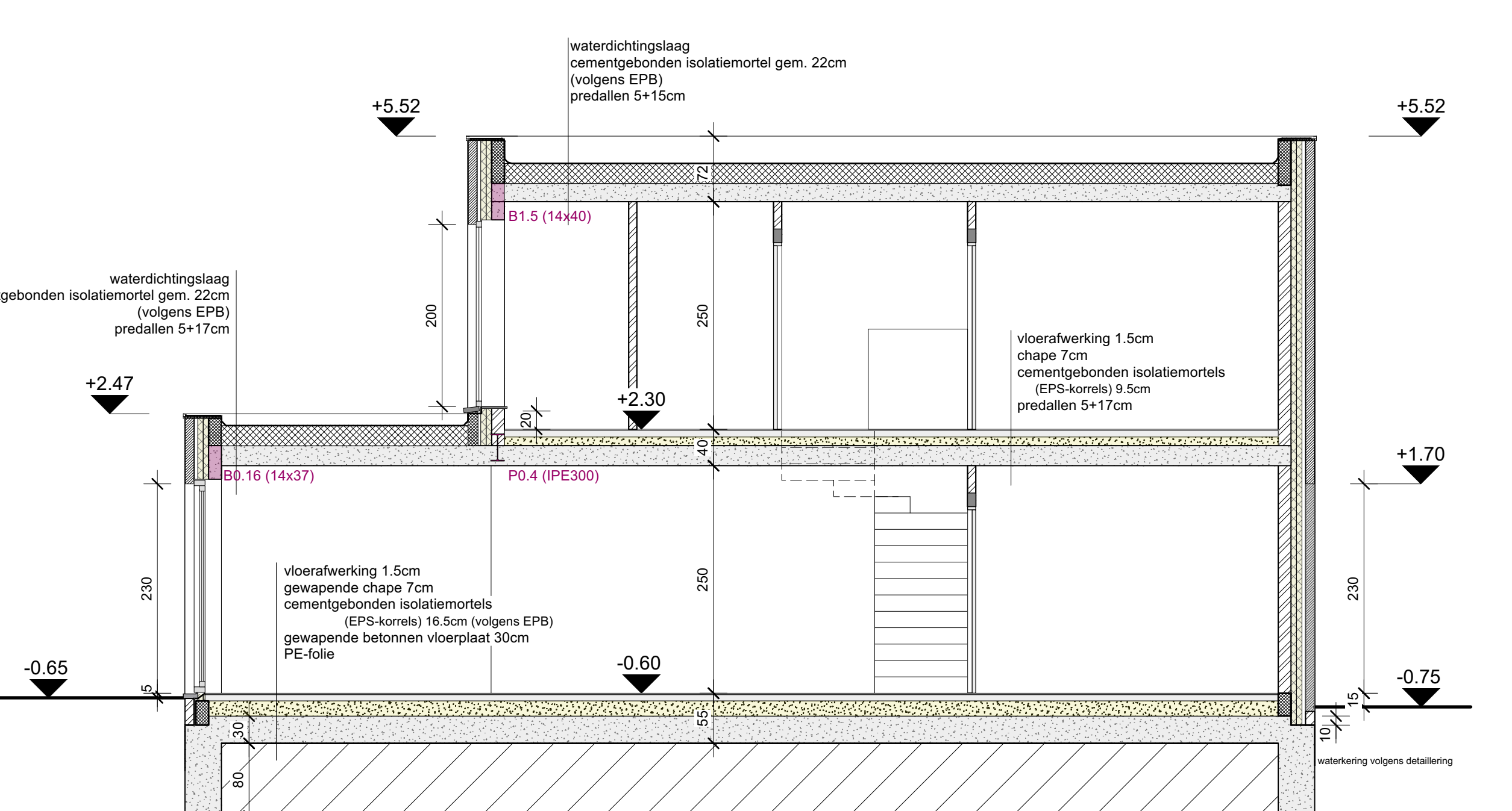
snede DD
