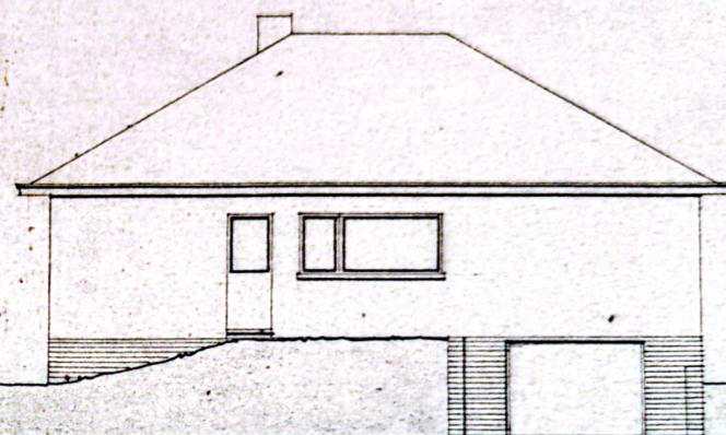
ACHTER GEVEL
