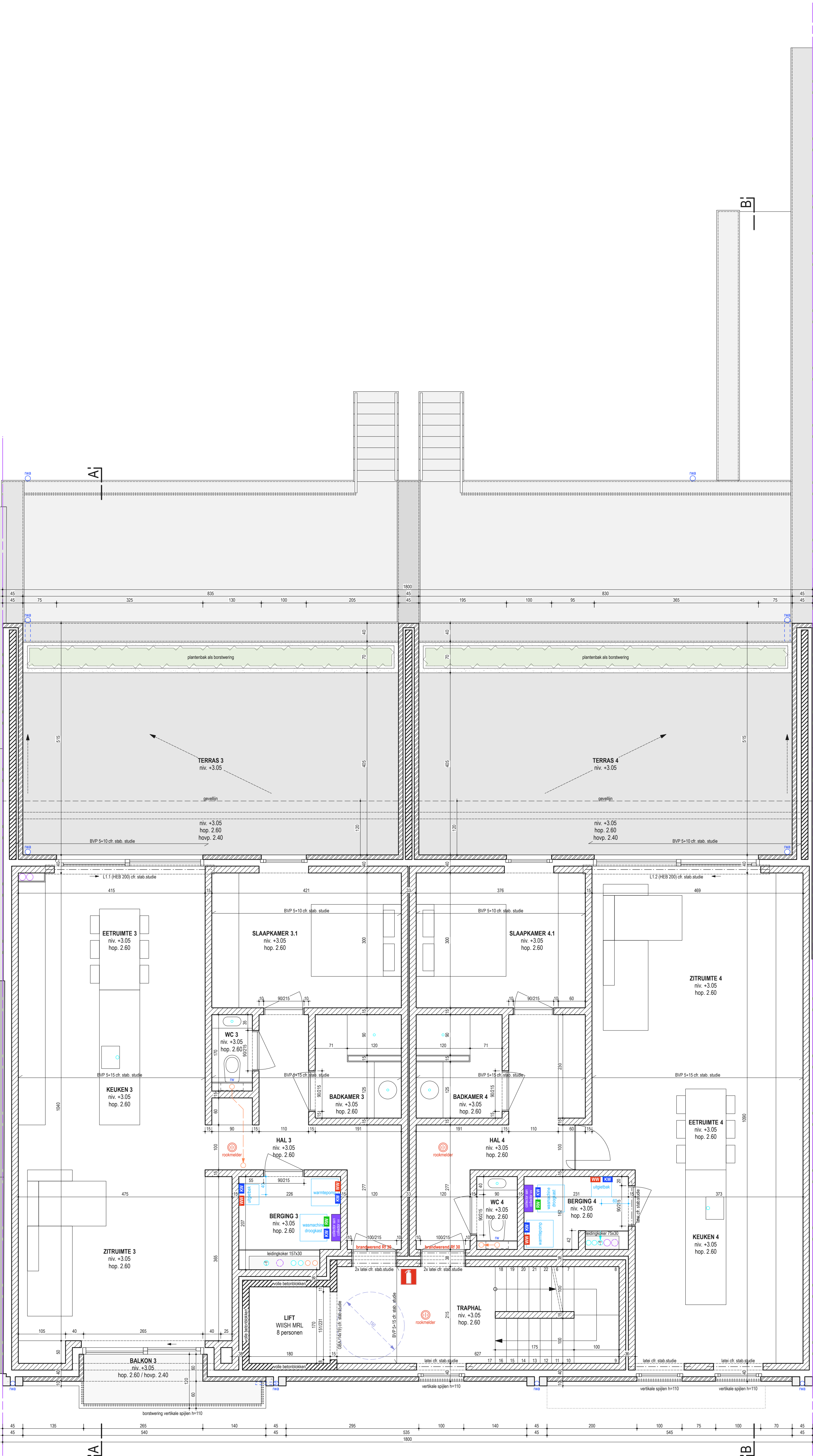
VERDIEPING 1 SCHAAL 1/50
