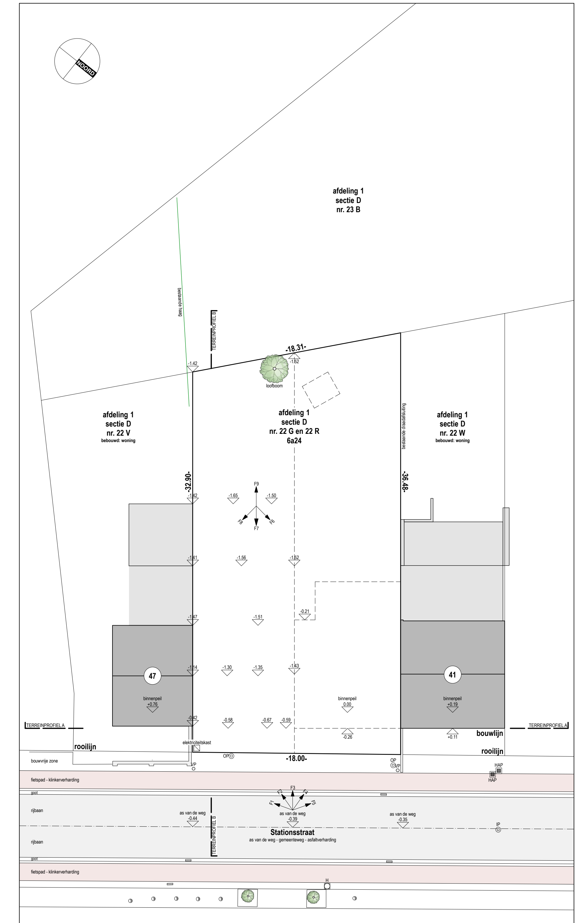
INPLANTINGSPLAN - TOESTAND NA AFBRAAK SCHAAL 1/200
