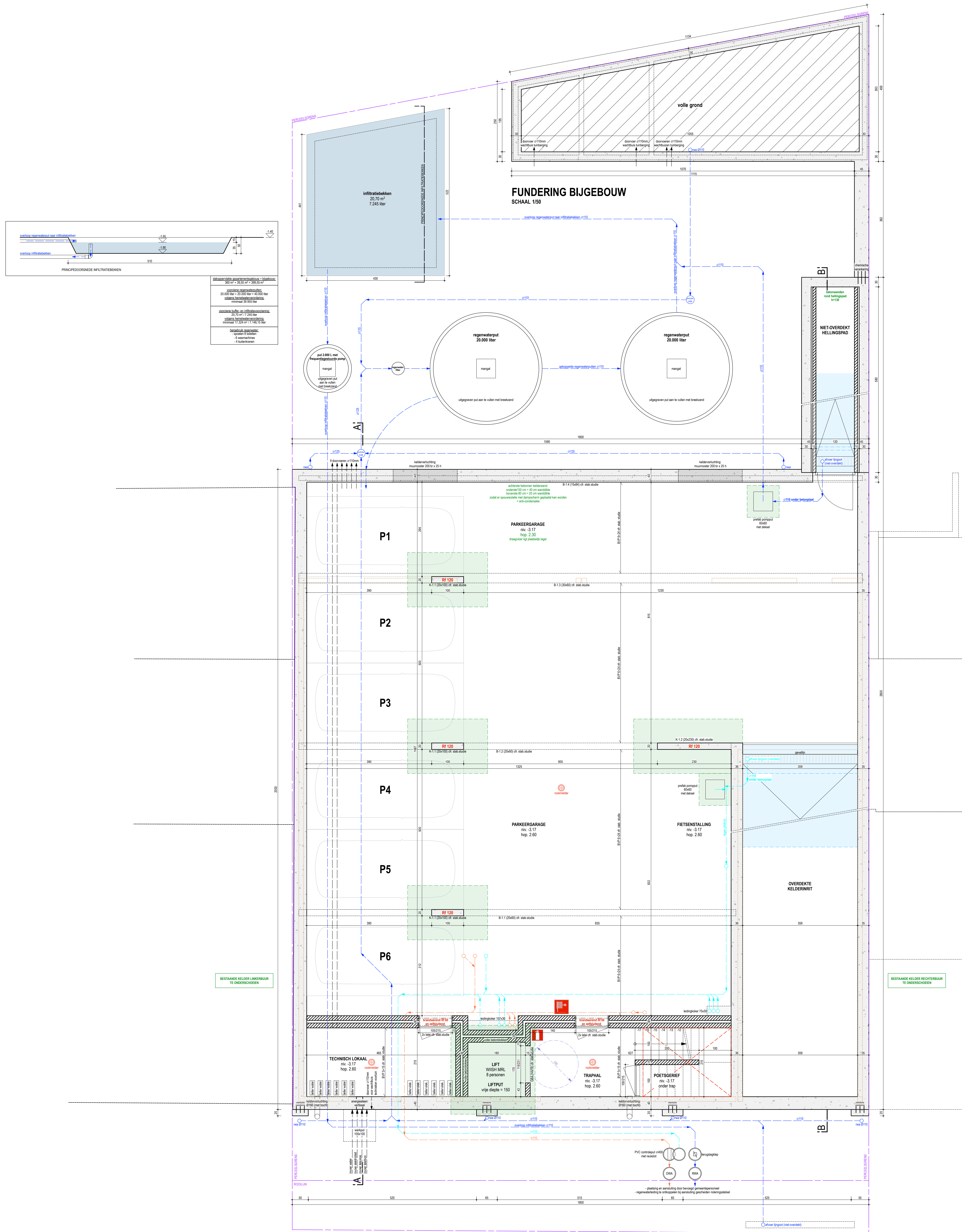
KELDER SCHEMATISCHE WEERGAVE VAN DE RIOLERING SCHAAL 1/50
