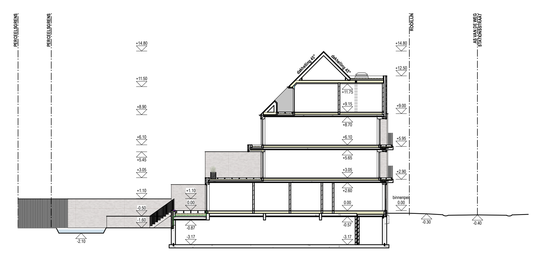
TERREINPROFIEL B SCHAAL 1/200
