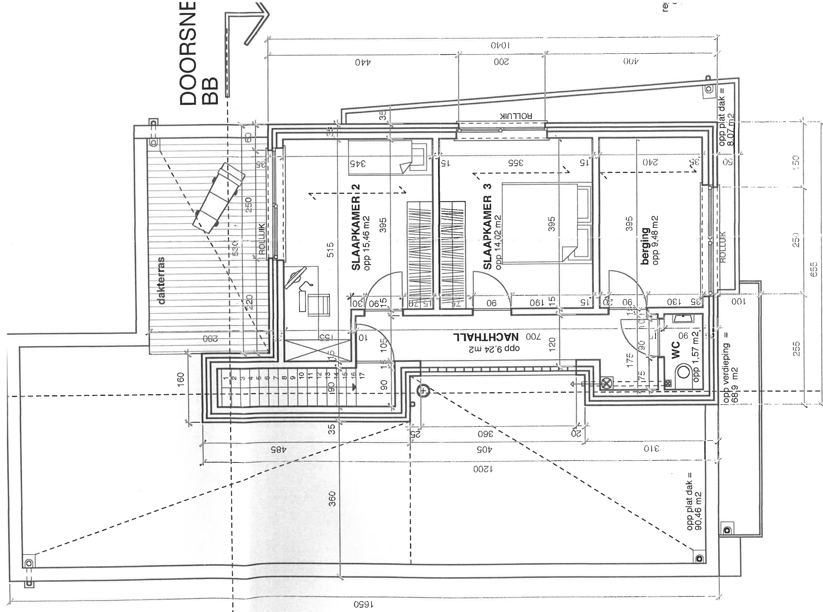
verdieping 1
