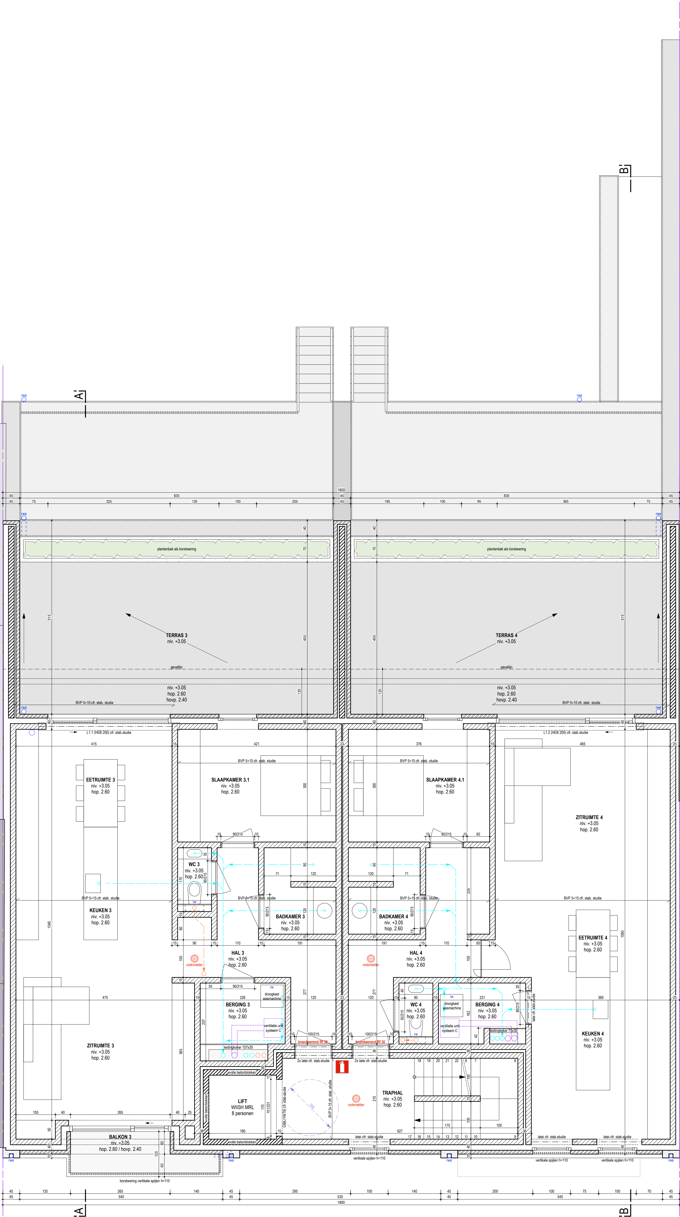
VERDIEPING 1 SCHAAL 1/50
