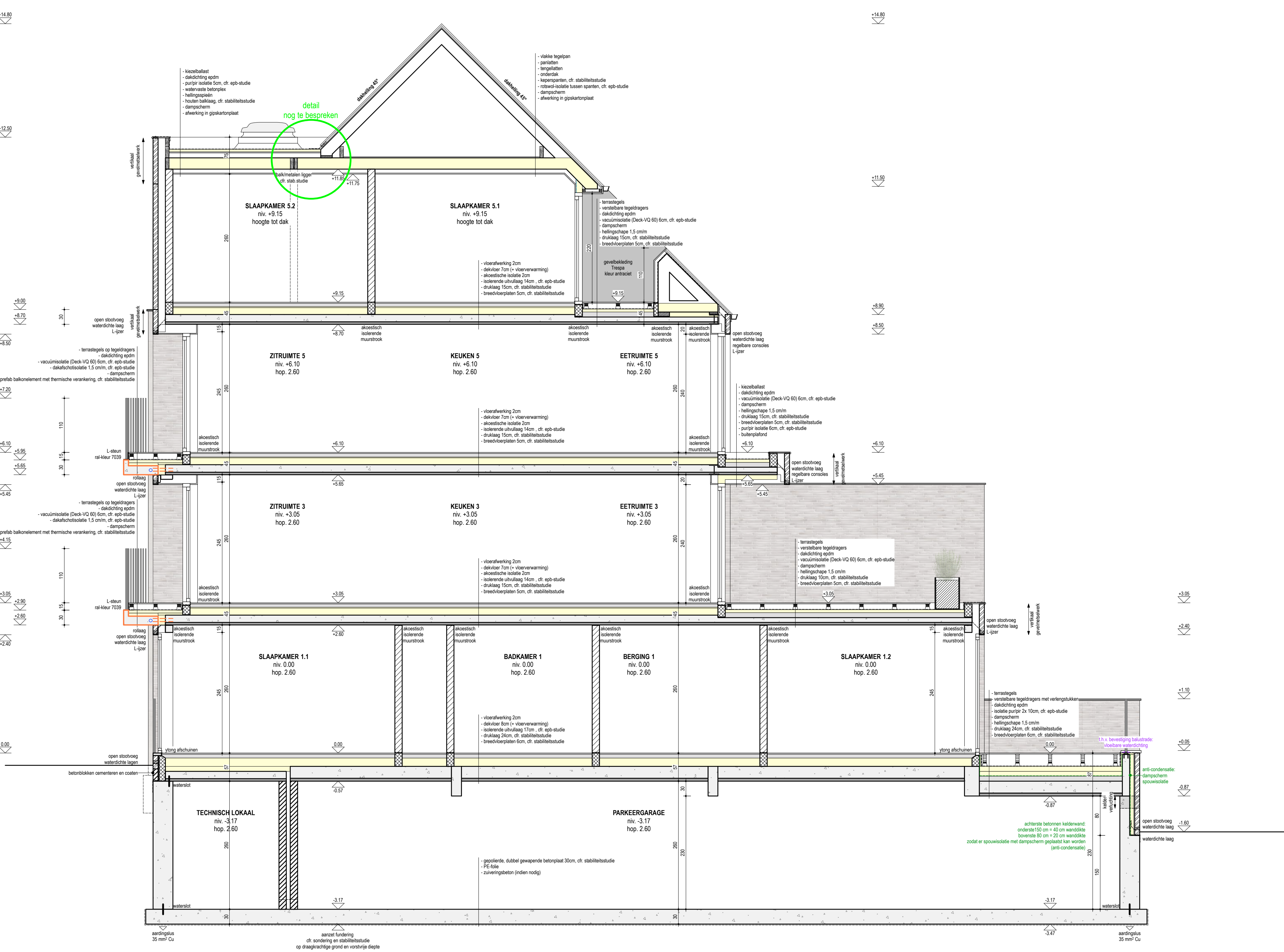
SNEDE AA SCHAAL 1/50
