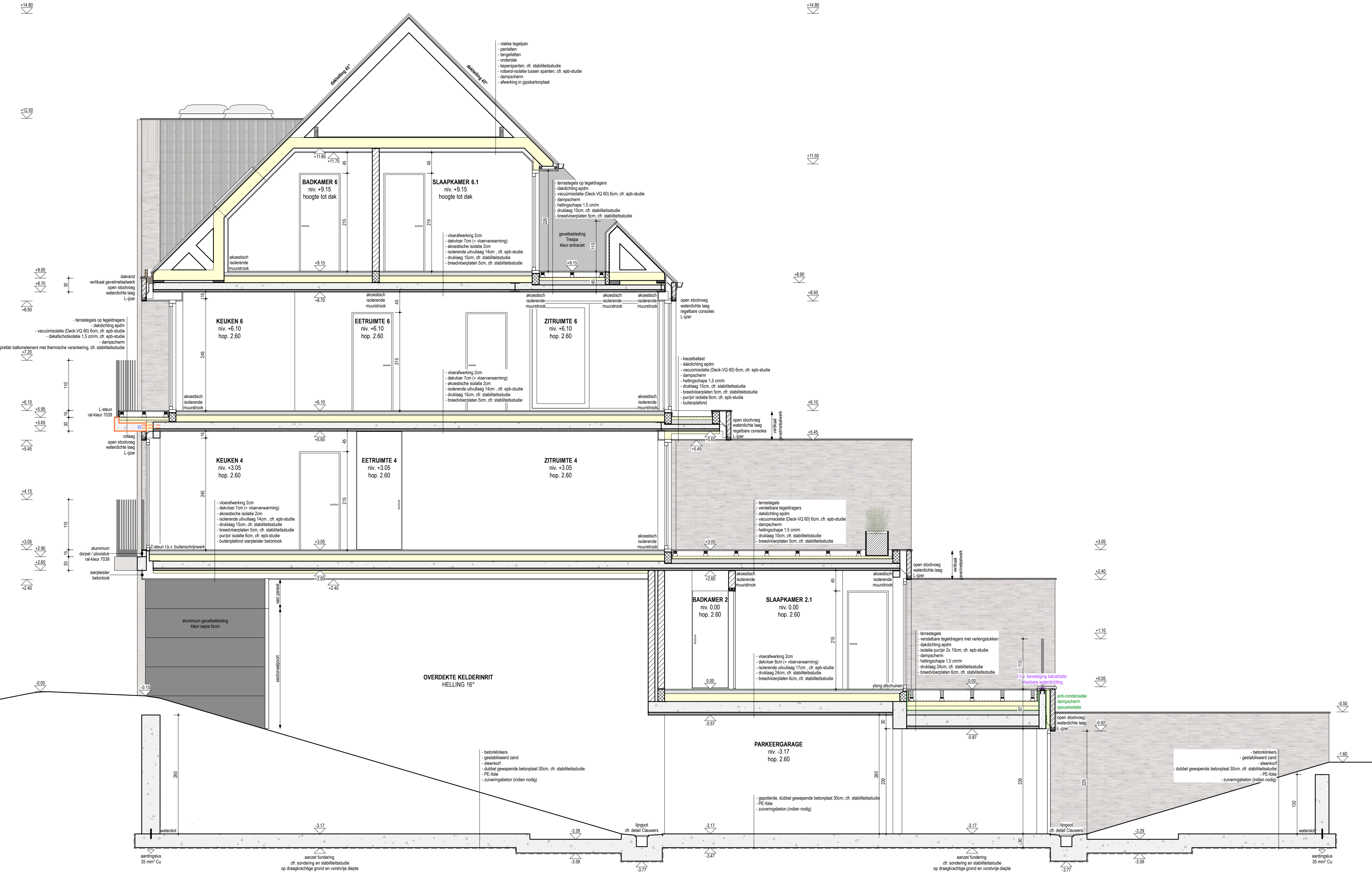
SNEDE BB SCHAAL 1/50
