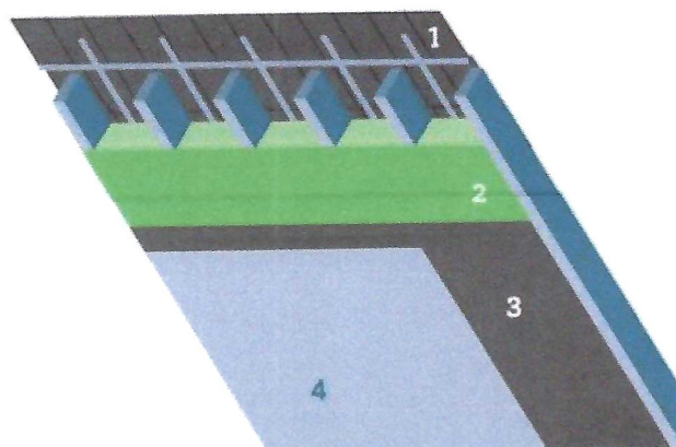
1. Onderdak | 2. Isolatie | 3. Damperscreen | 4. binnenafwerking
