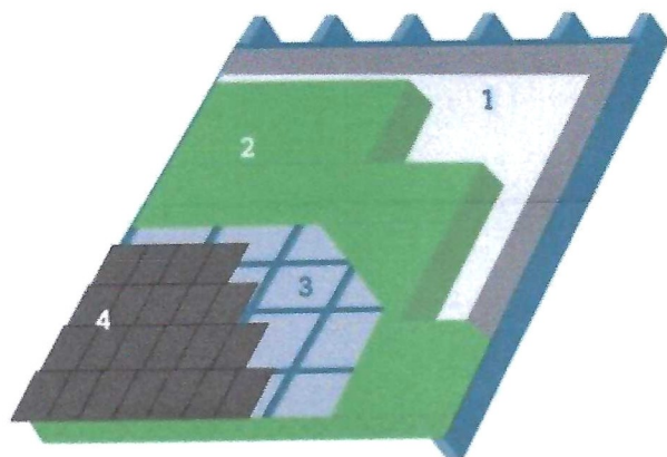
1. Damperscreen | 2. Isolatie | 3. Onderdak | 4. Dakbekleding
