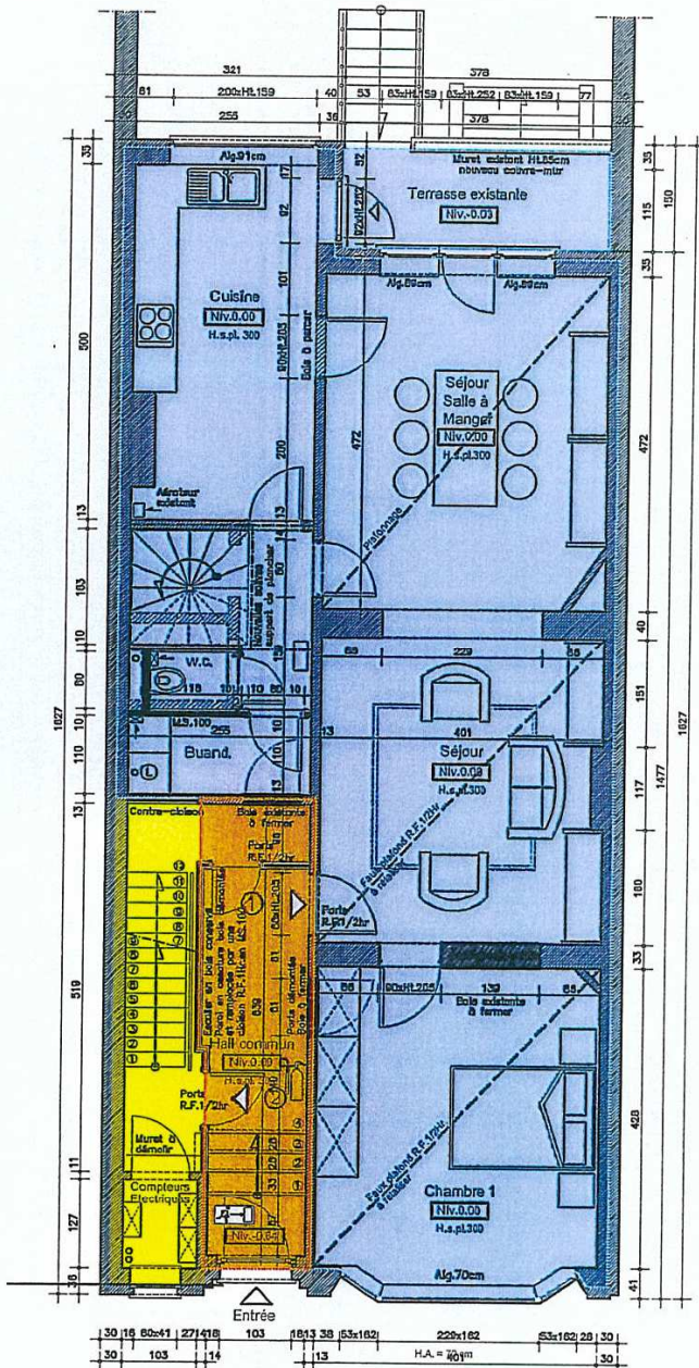
PLAN DU REZ-DE-CHAUSSEE
