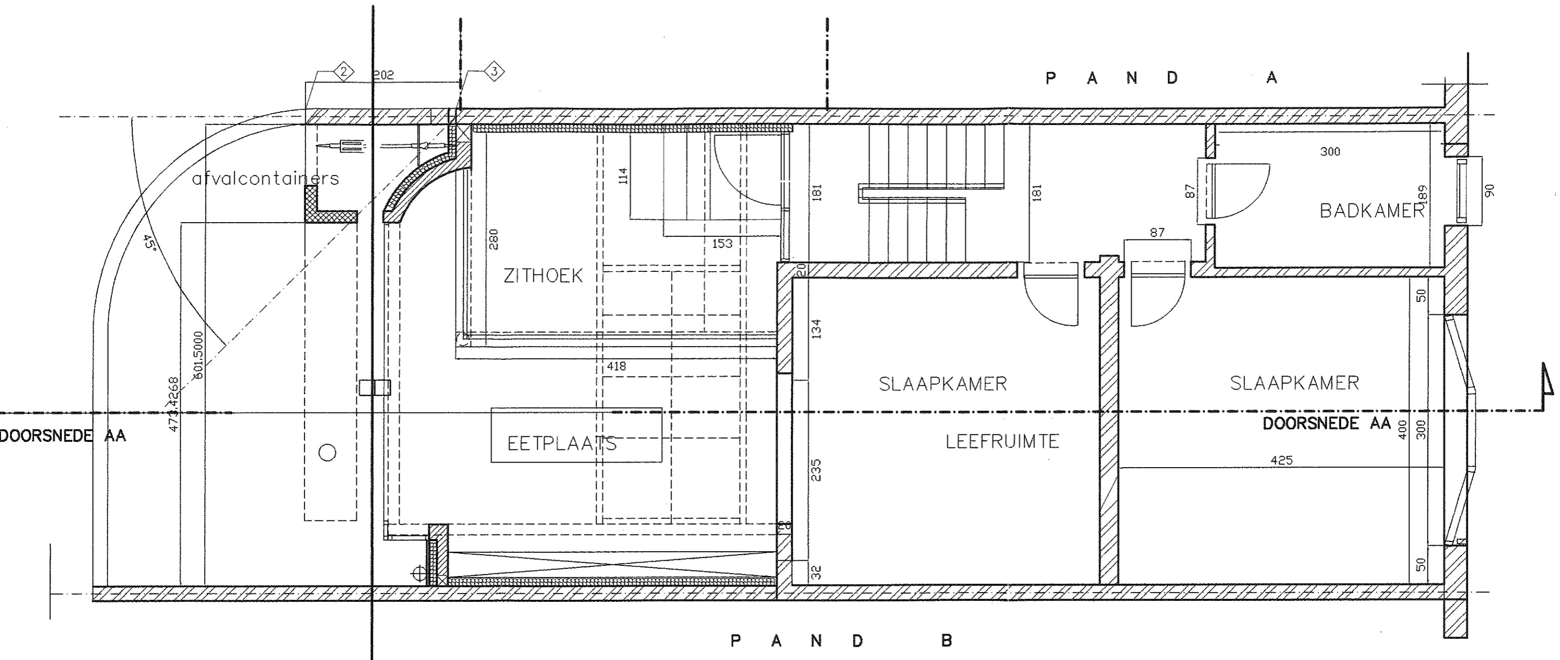
1 STE VERDIEPING NA VERBOUWING
