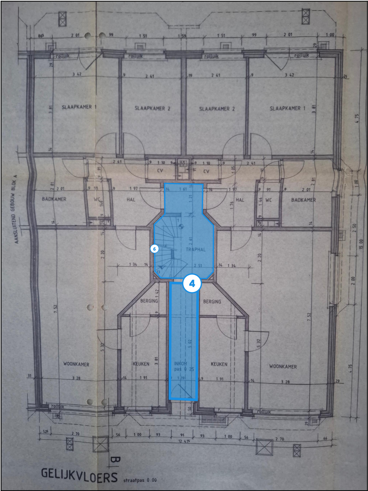
Legende van plan 2.3: Gelijkvloers plafond
