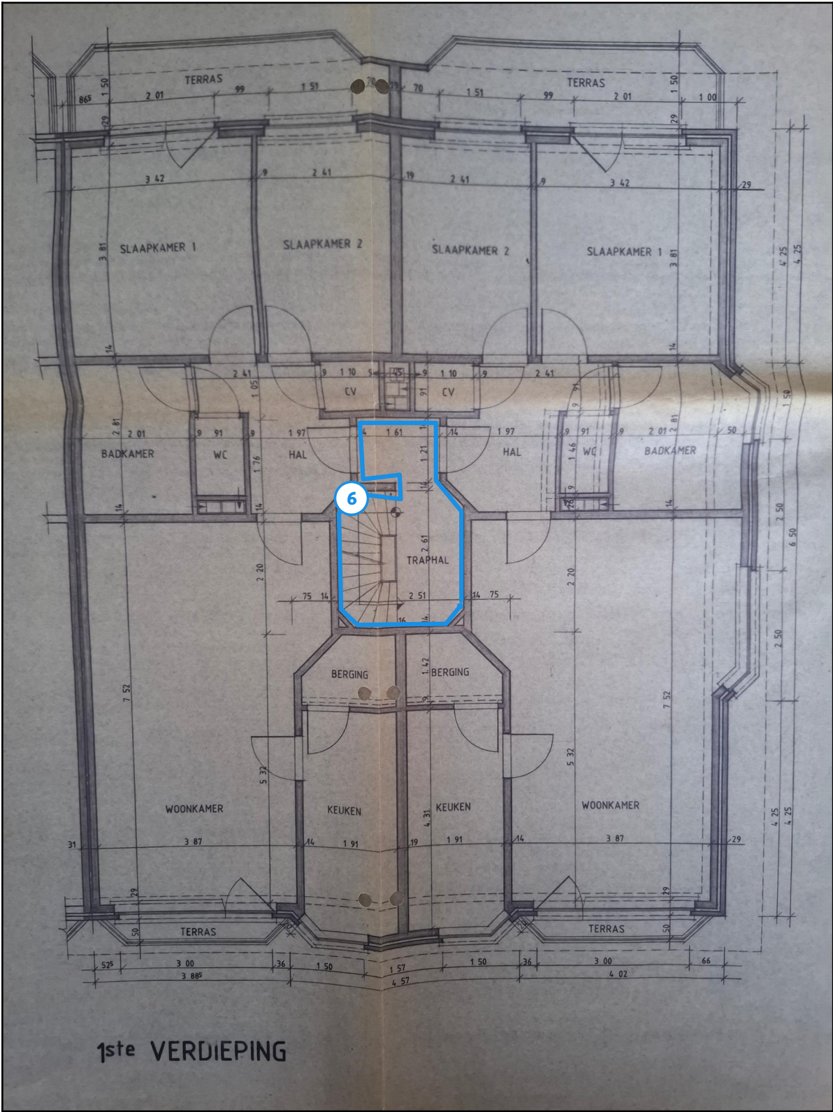
Legende van plan 2.4: Verdieping 1
