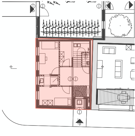
Grondplan
