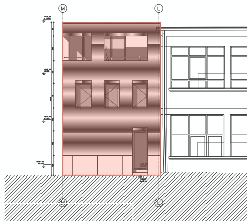
Gevel Z-O
