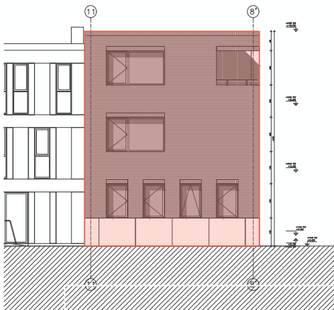
Gevel Z-W
