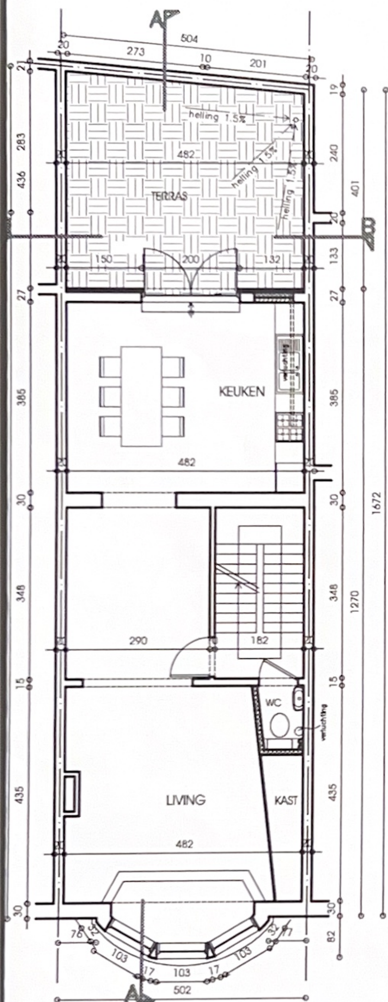
VERDIEPING 1
