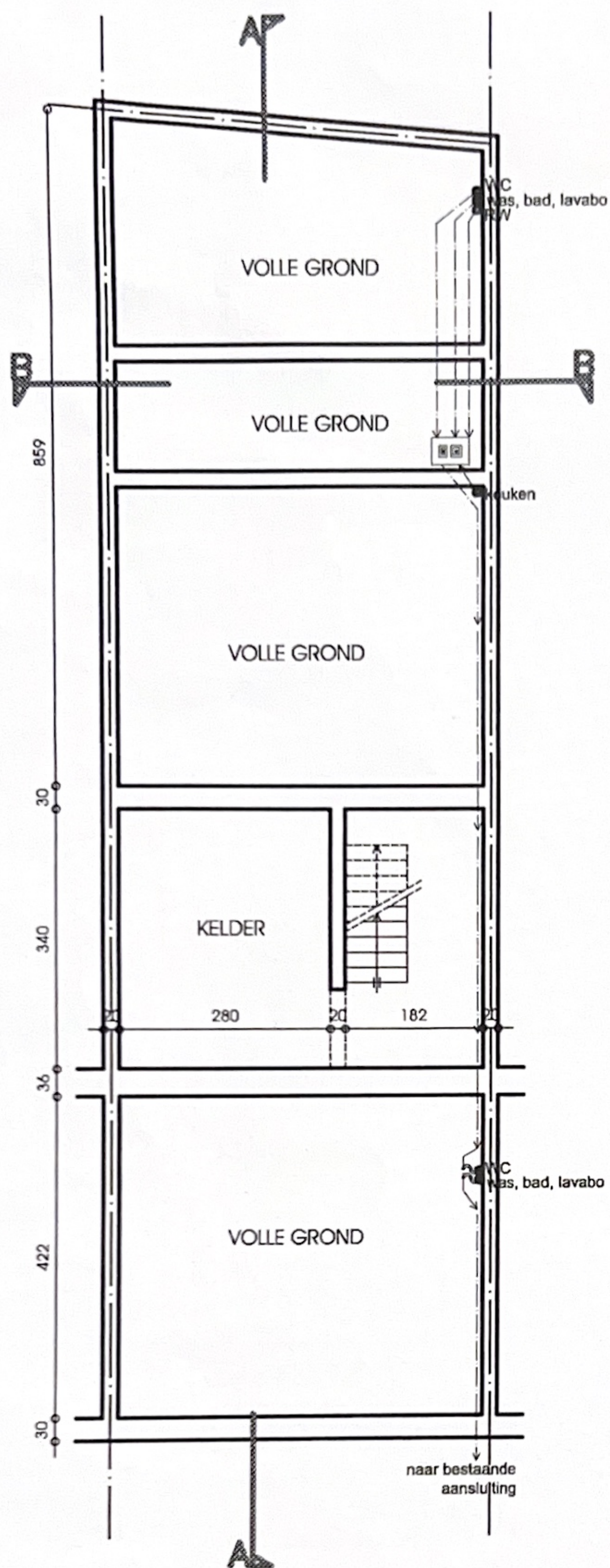
KELDER (ONGEWIJZIGD)
