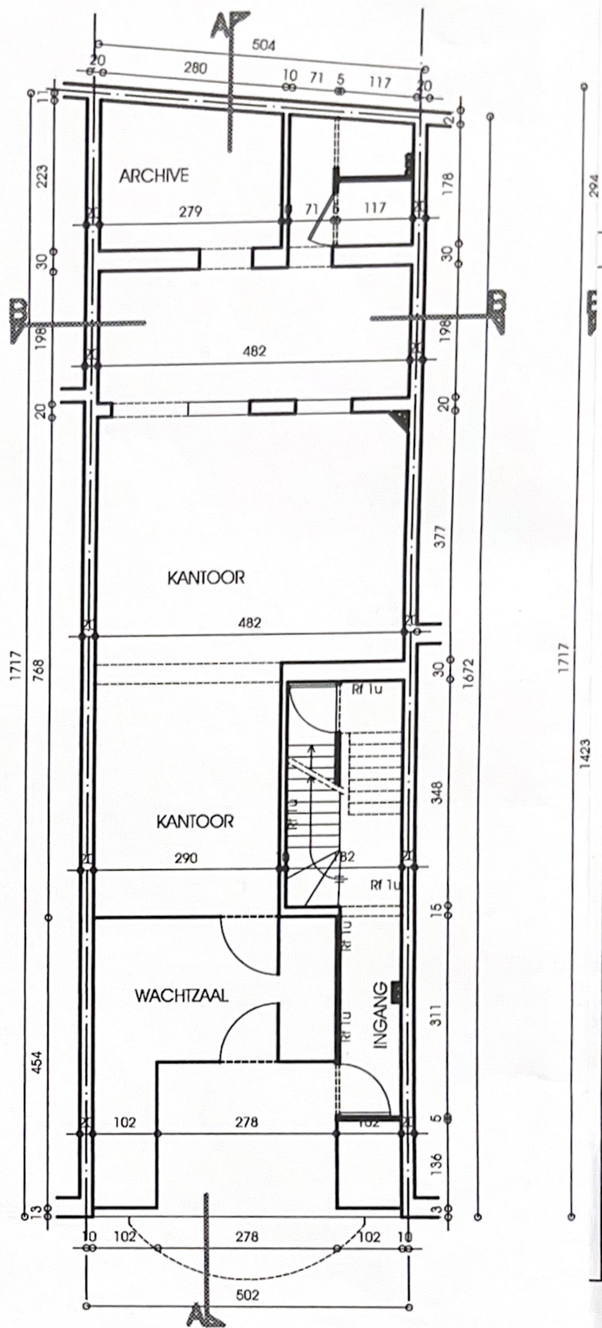
GELIJKVLOERS (ONGEWIJZIGD)
