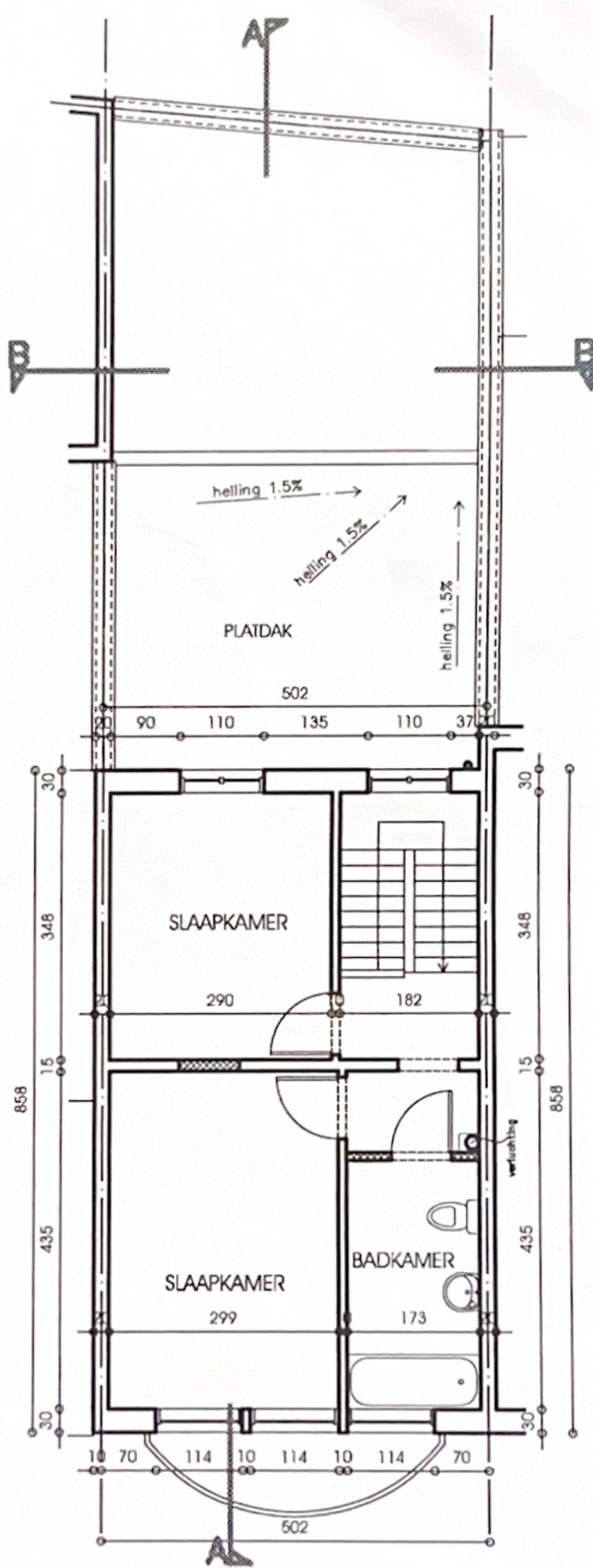
VERDIEPING 2
