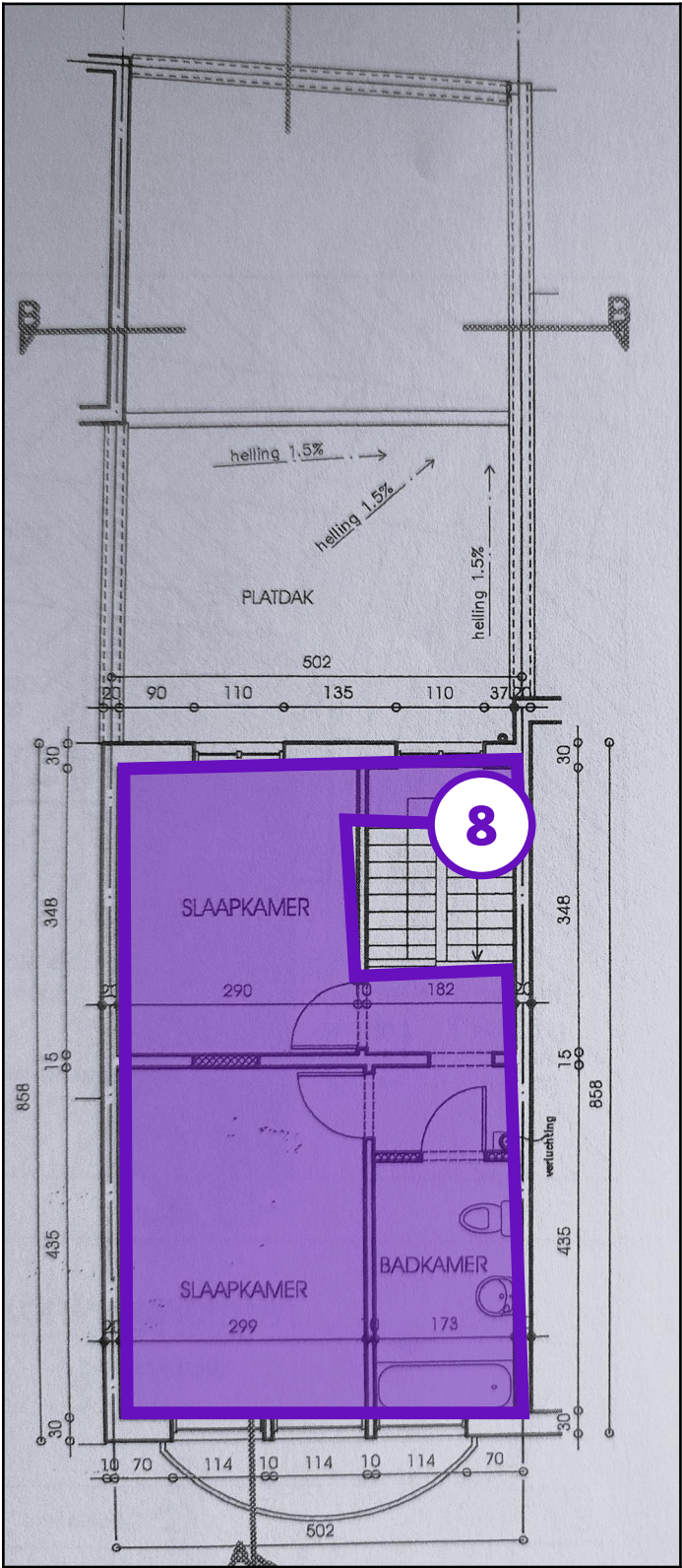
Legende van plan 1.10: vloerplan v+2
