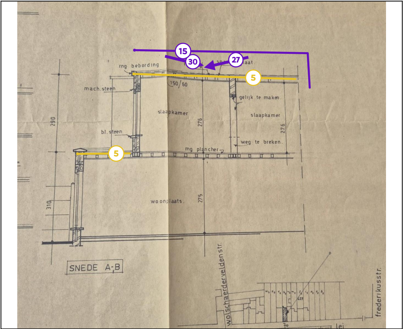
Legende van plan 1.6: Snede
