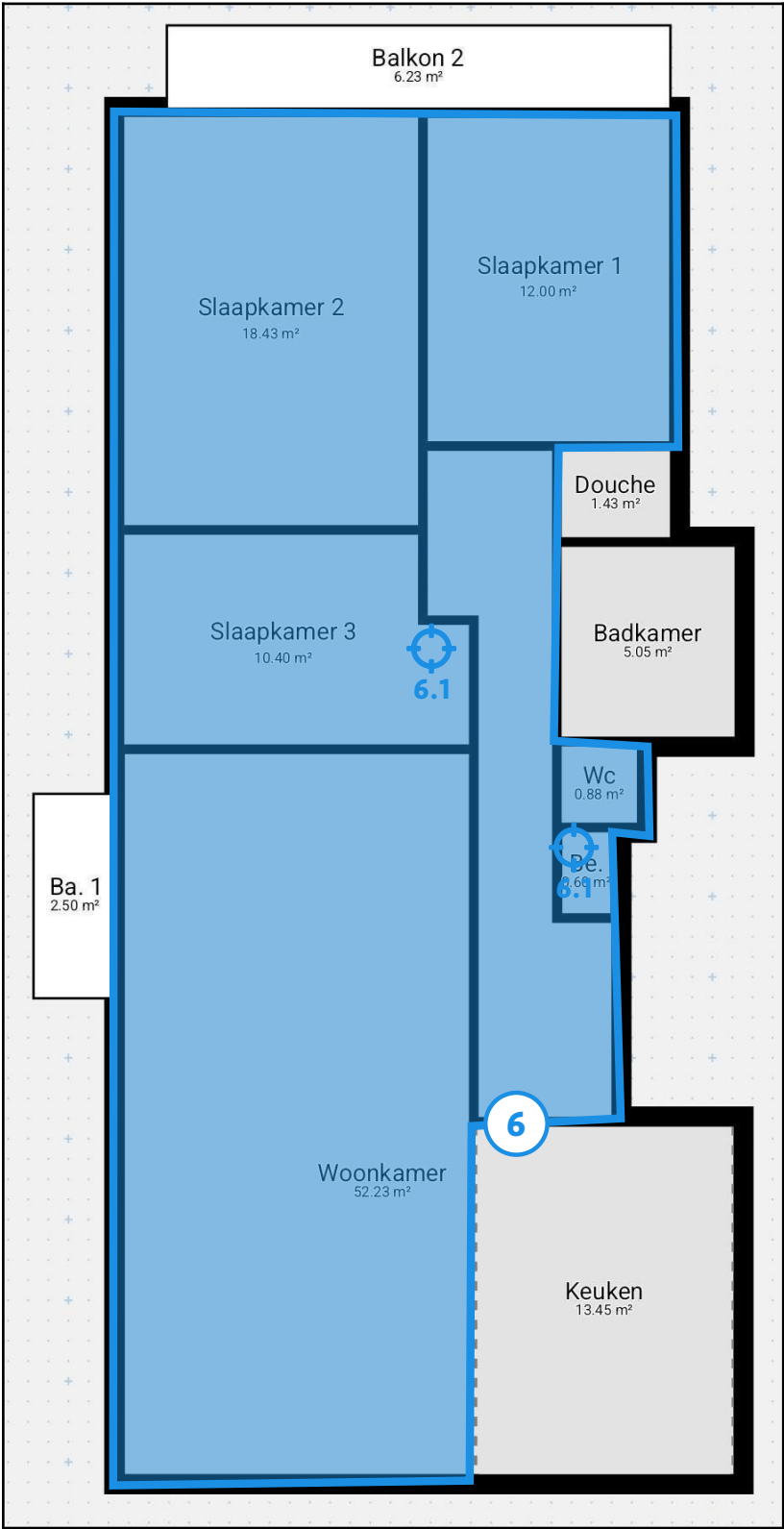
Legende van plan 1.3: Appartement 402
