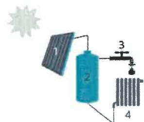
1 Zonnecollector | 2 Opslagvat zonneboiler | 3 Sanitair warm water | 4 Aangerechtigd voor ruimteverwarming (optioneel)
