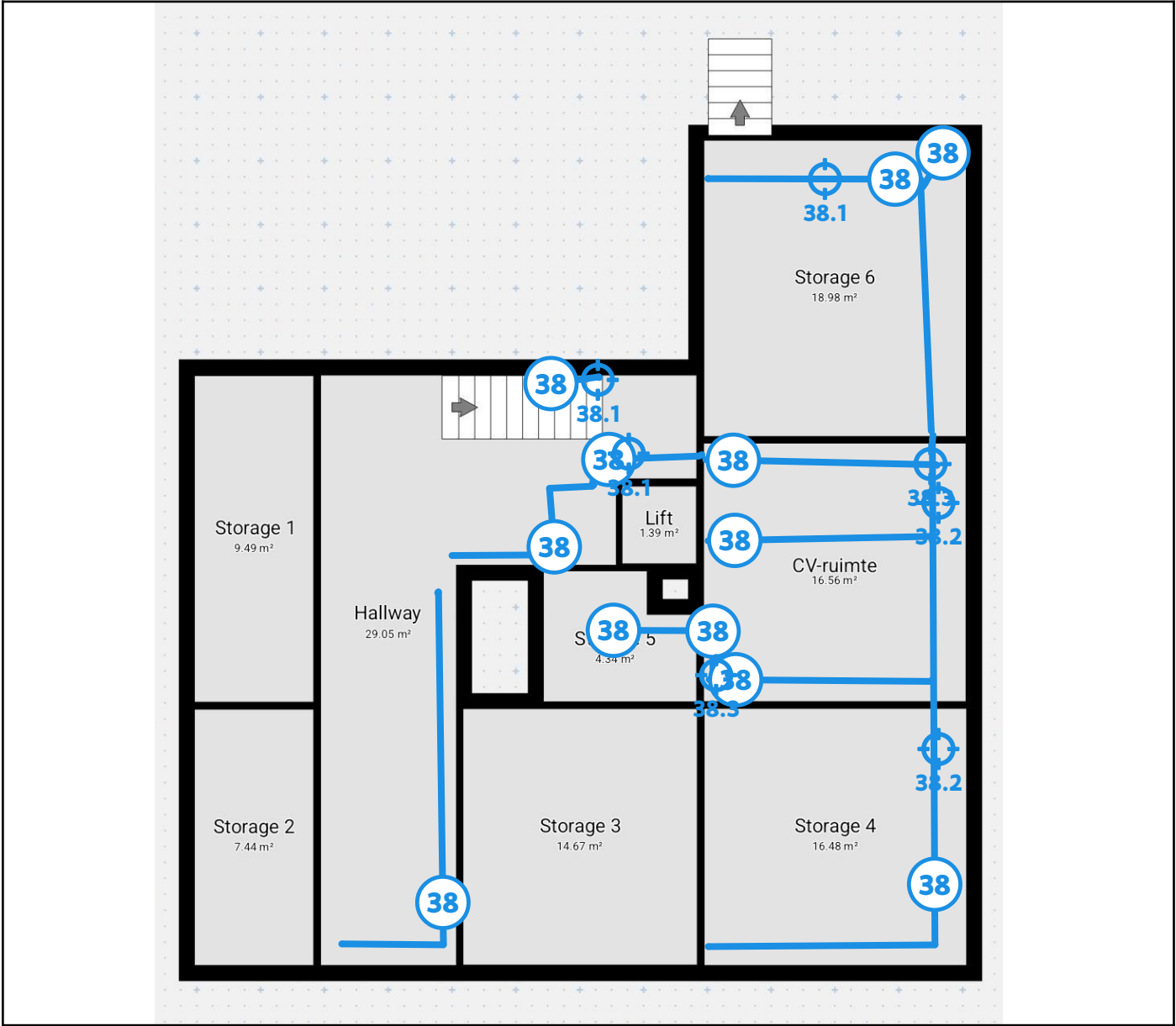
Legende van plan 1.3: Kelder
