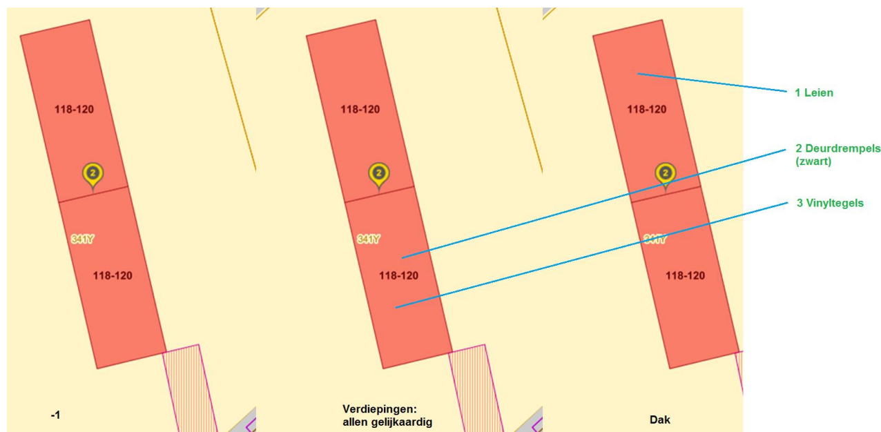
Figuur 2: Staalnameplan (geen detailplan beschikbaar): asbesthoudende materialen worden rood aangeduid, mogelijk asbesthoudende materialen oranje, asbestvrije materialen in groen.
