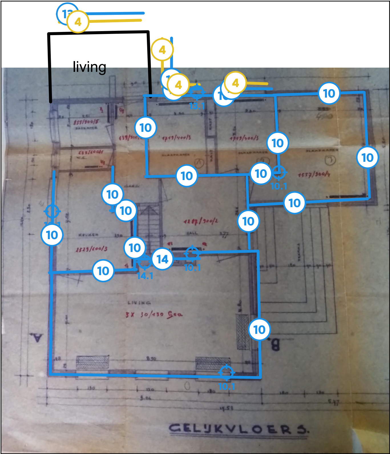
Legende van plan 1.2: Gelijkvloers. Pleisterwerk muren, kit,mastiek
