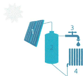
1. Zonnecollector | 2. Opslagvat zonneboiler | 3. Sanitair warm water | 4. Afgevoerd warmte voor verwarming of ruimteverwarming
