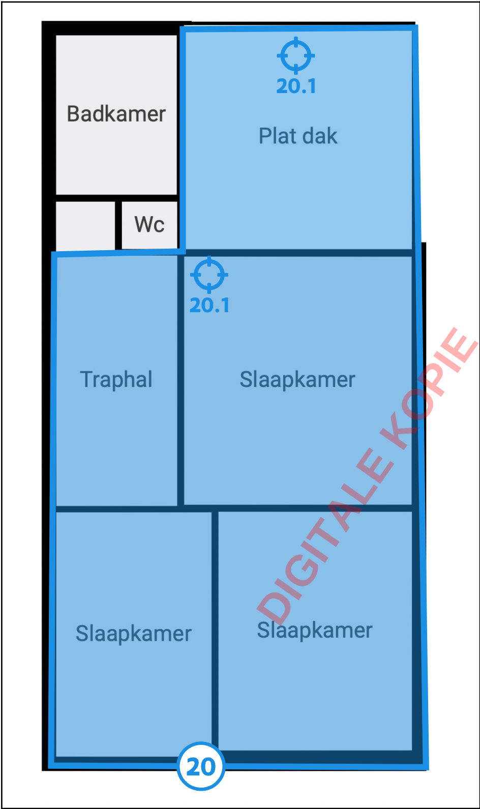
Legende van plan 1.7: Grondplan - Verdieping
