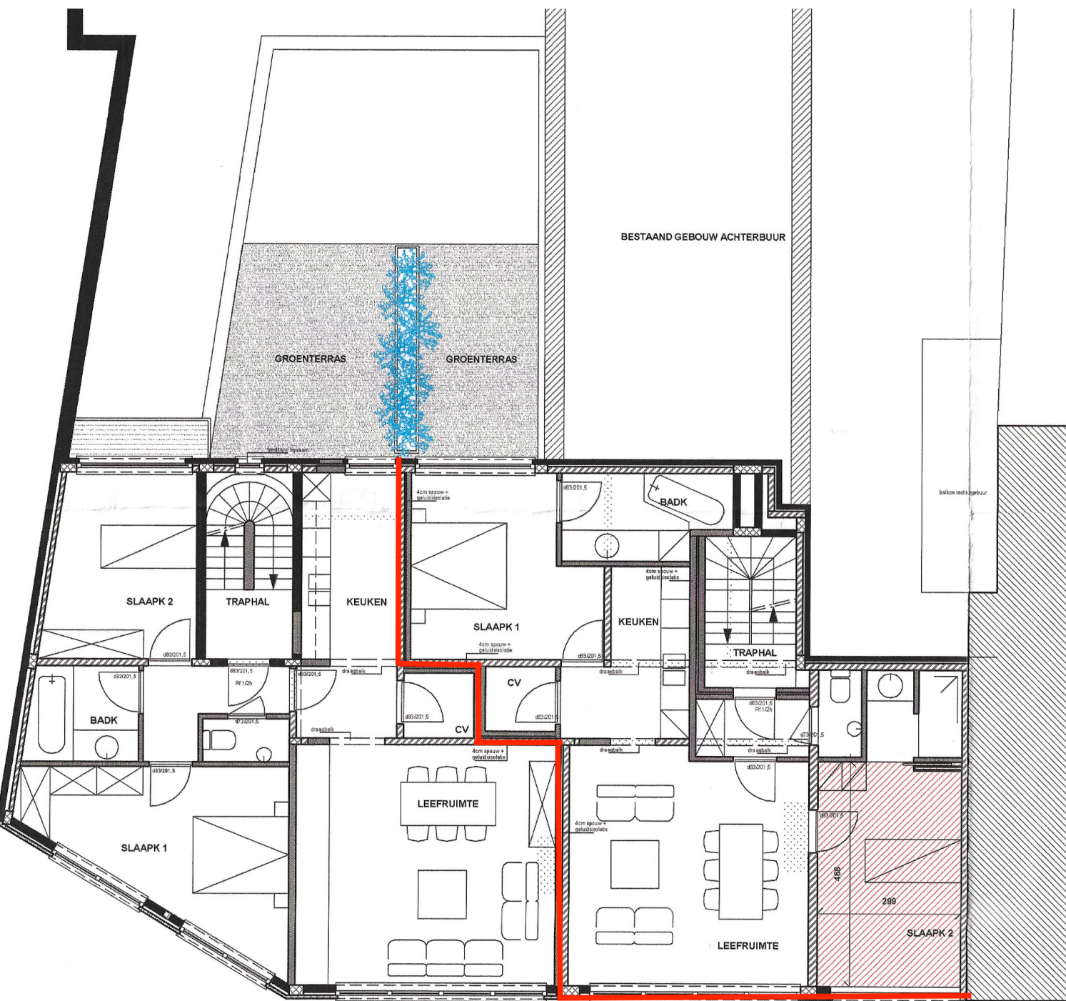
1° VERDIEPINGSPLAN 1/100
