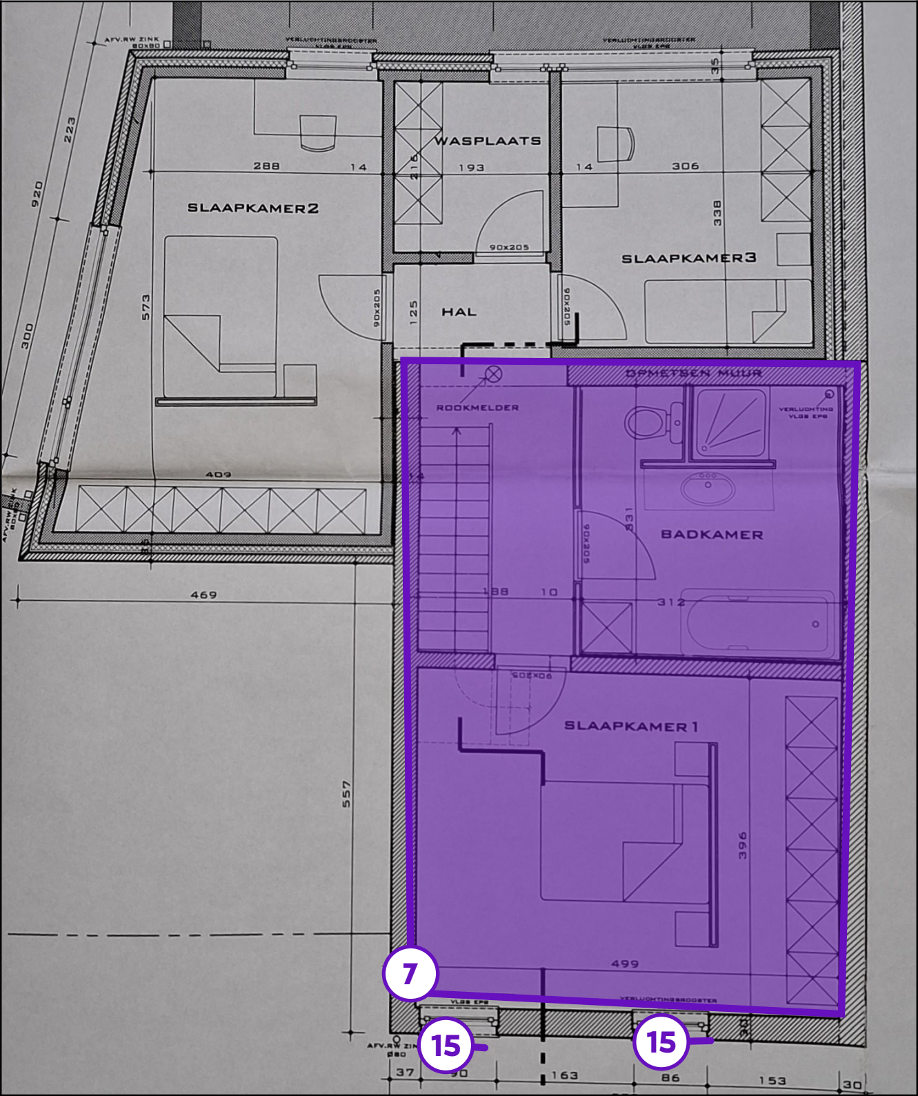
Legende van plan 1.8: Verdiep 1 deel 2
