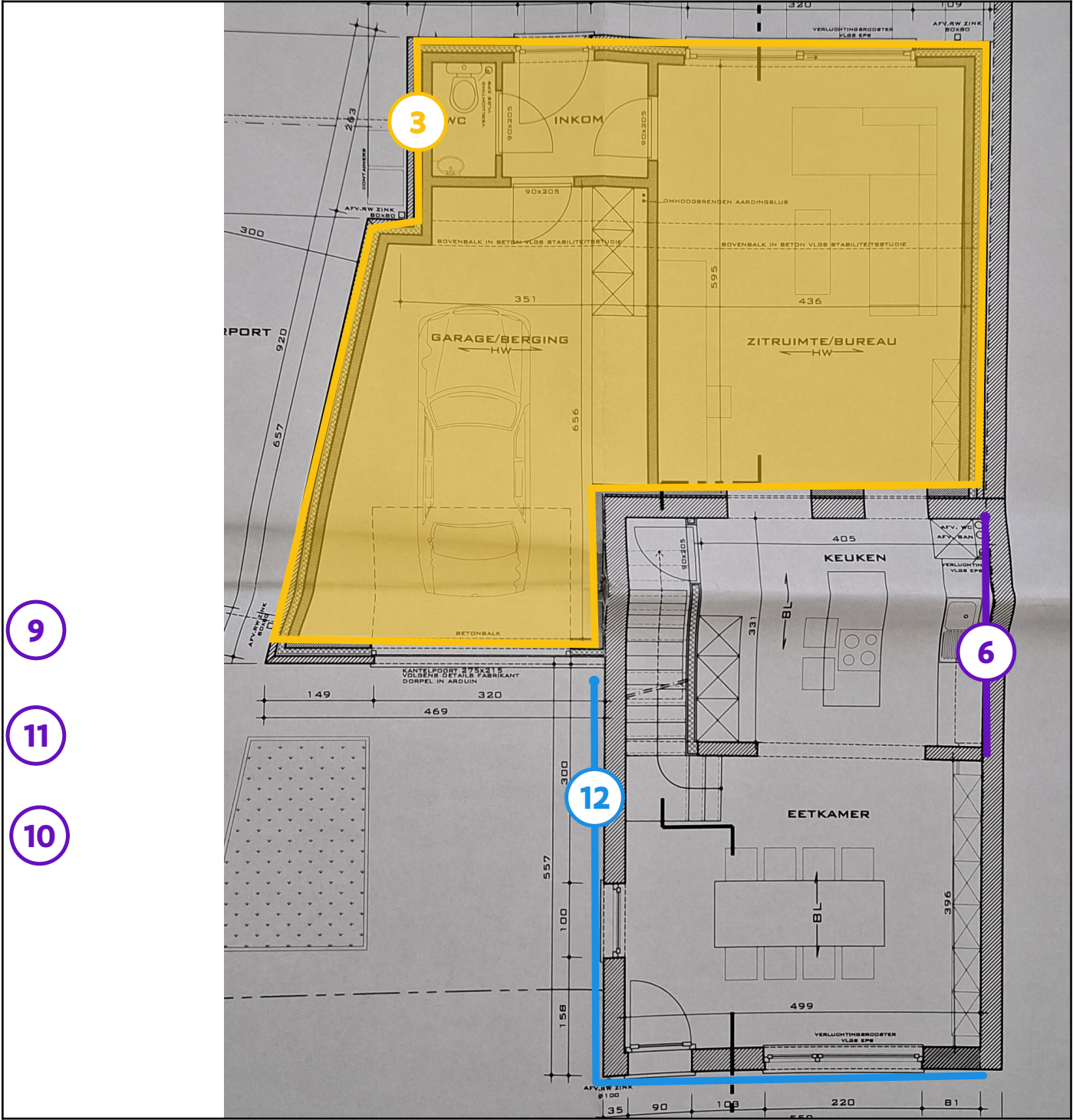
Legende van plan 1.3: GVL deel 1
