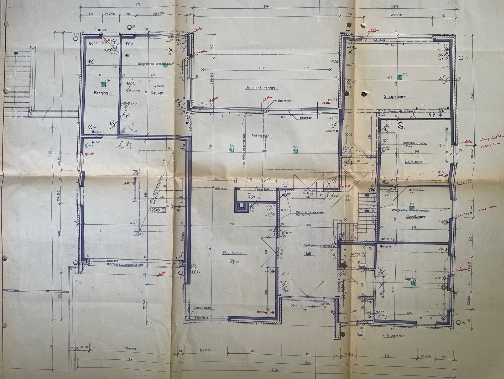
Plan gelijkvloers
