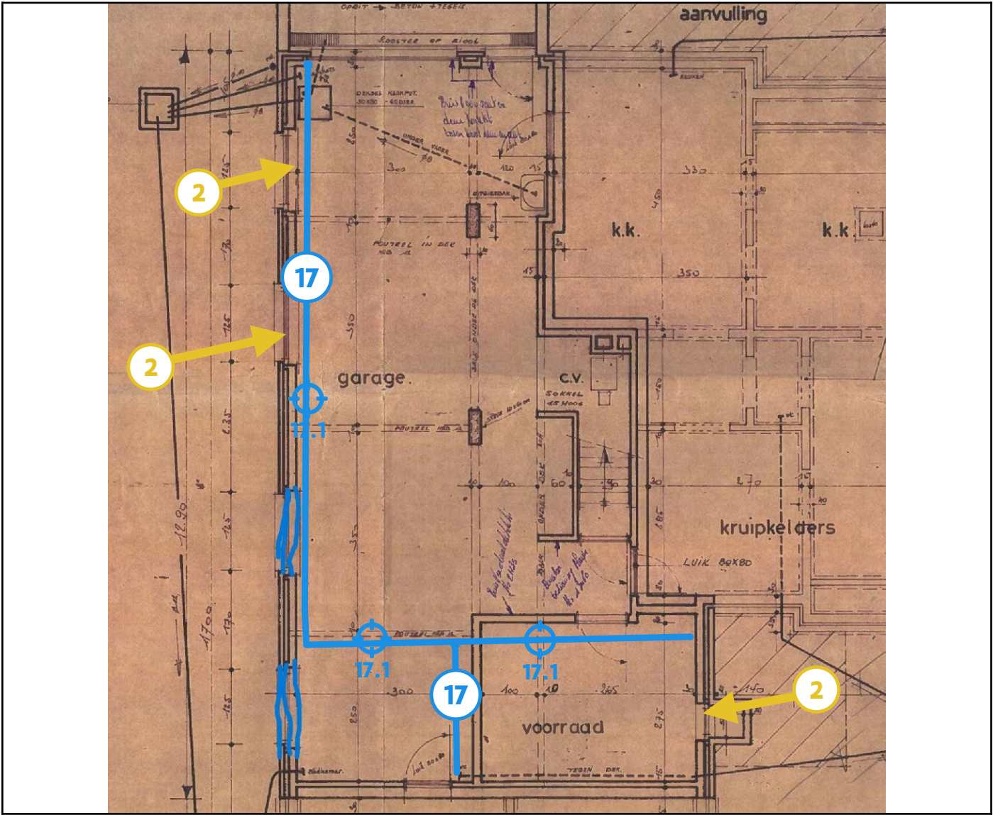
Legende van plan 1.5: kelder verdieping
