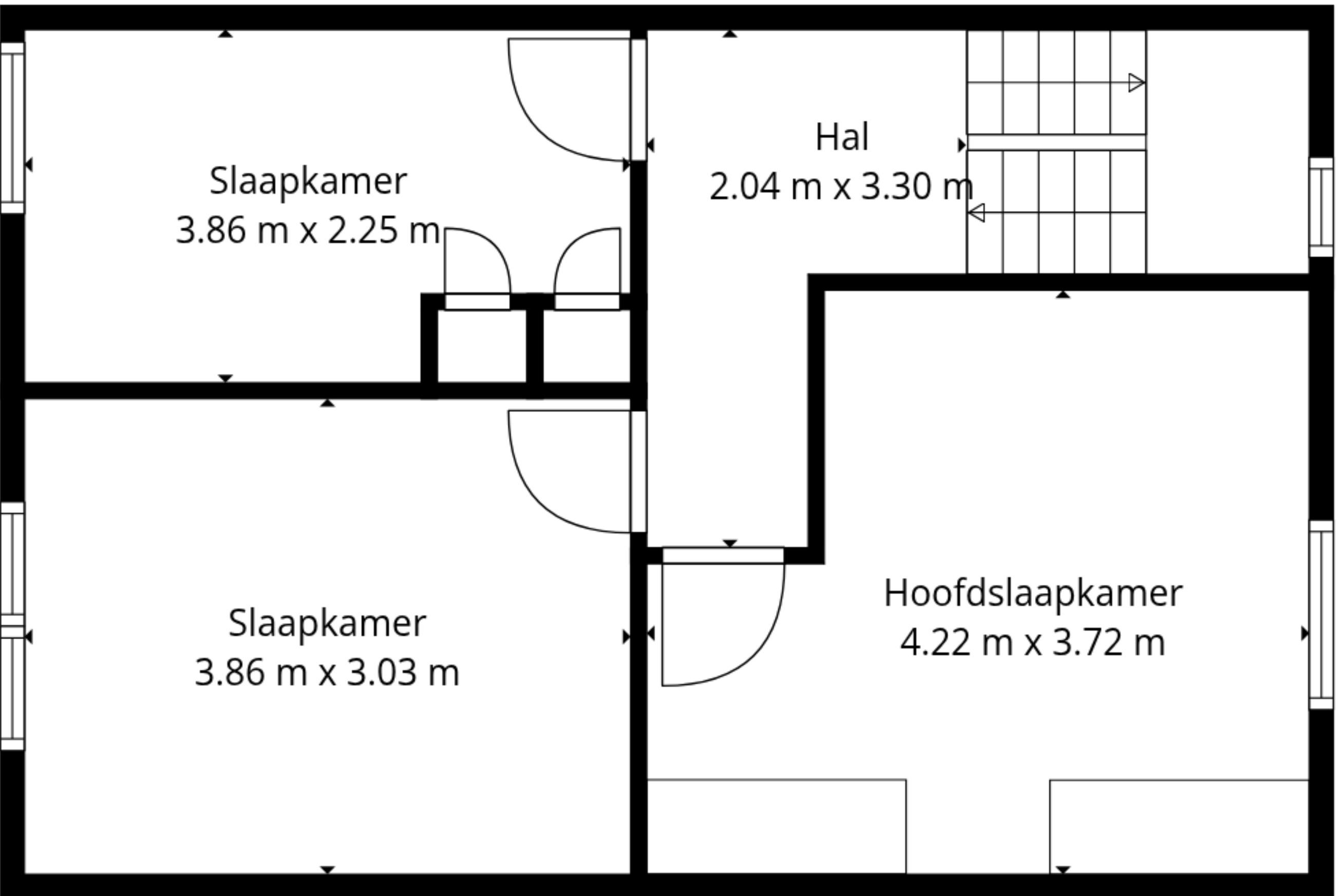
1e Verdieping
