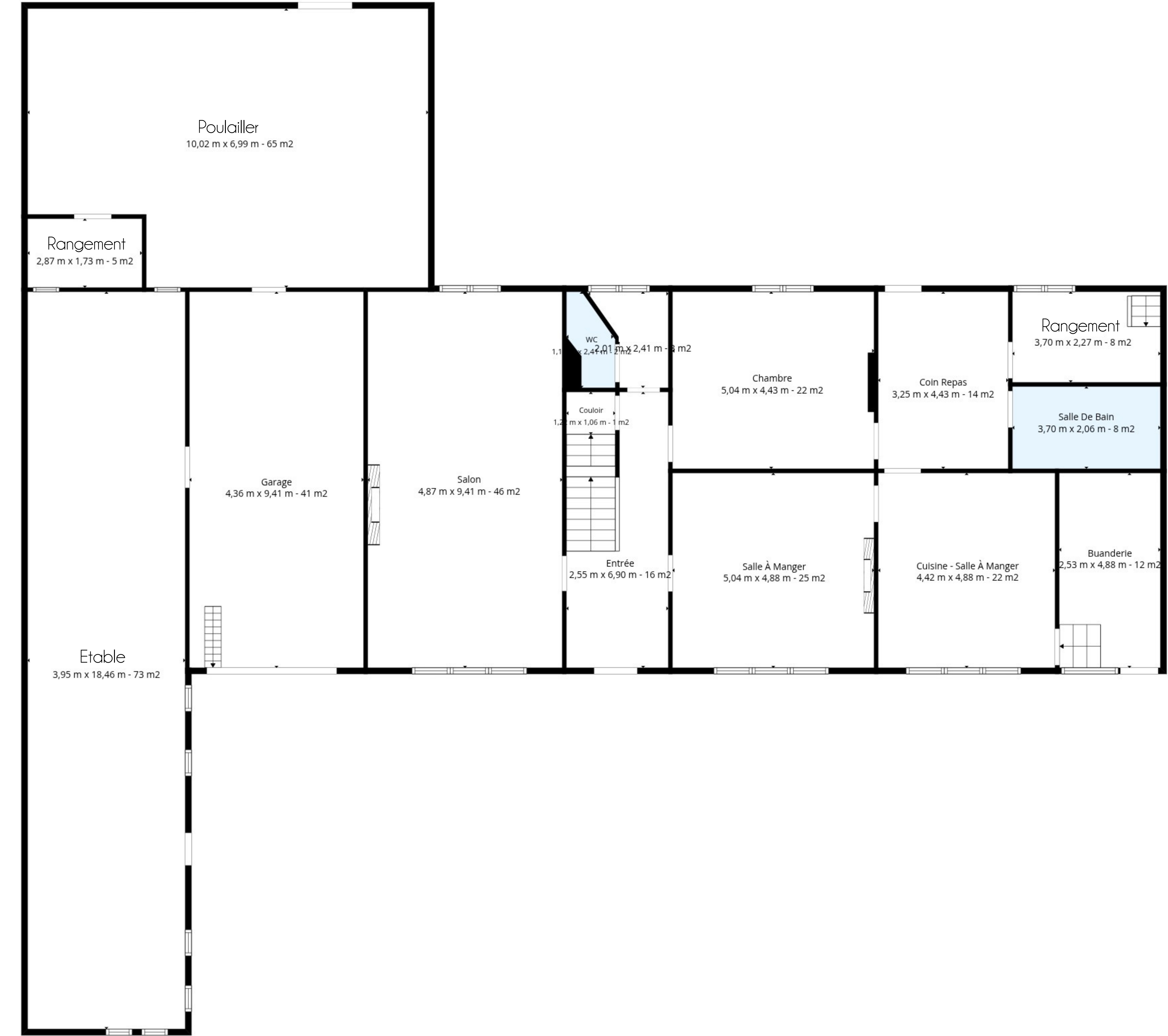
Rez-de-chaussée
