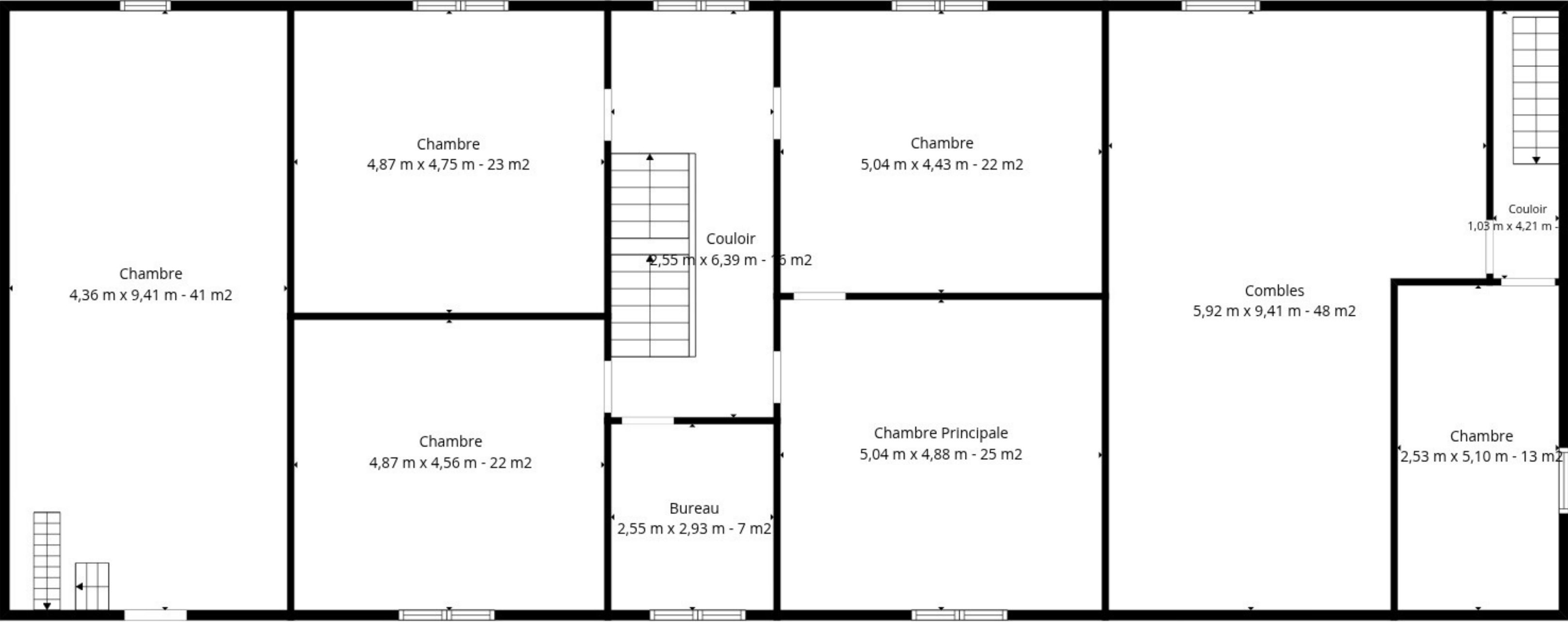
1er Étage
