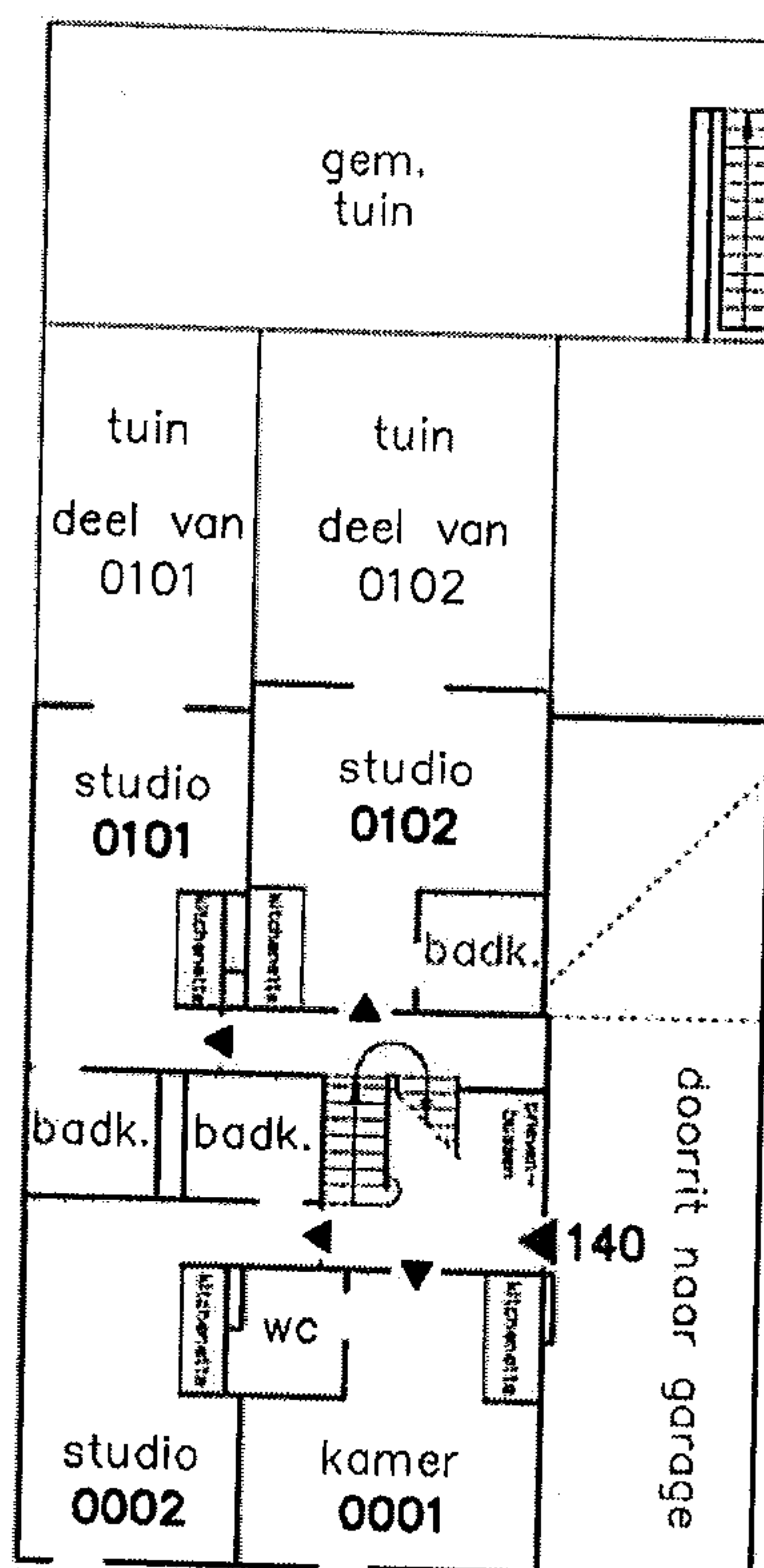
Parkstraat gelijkvloers
