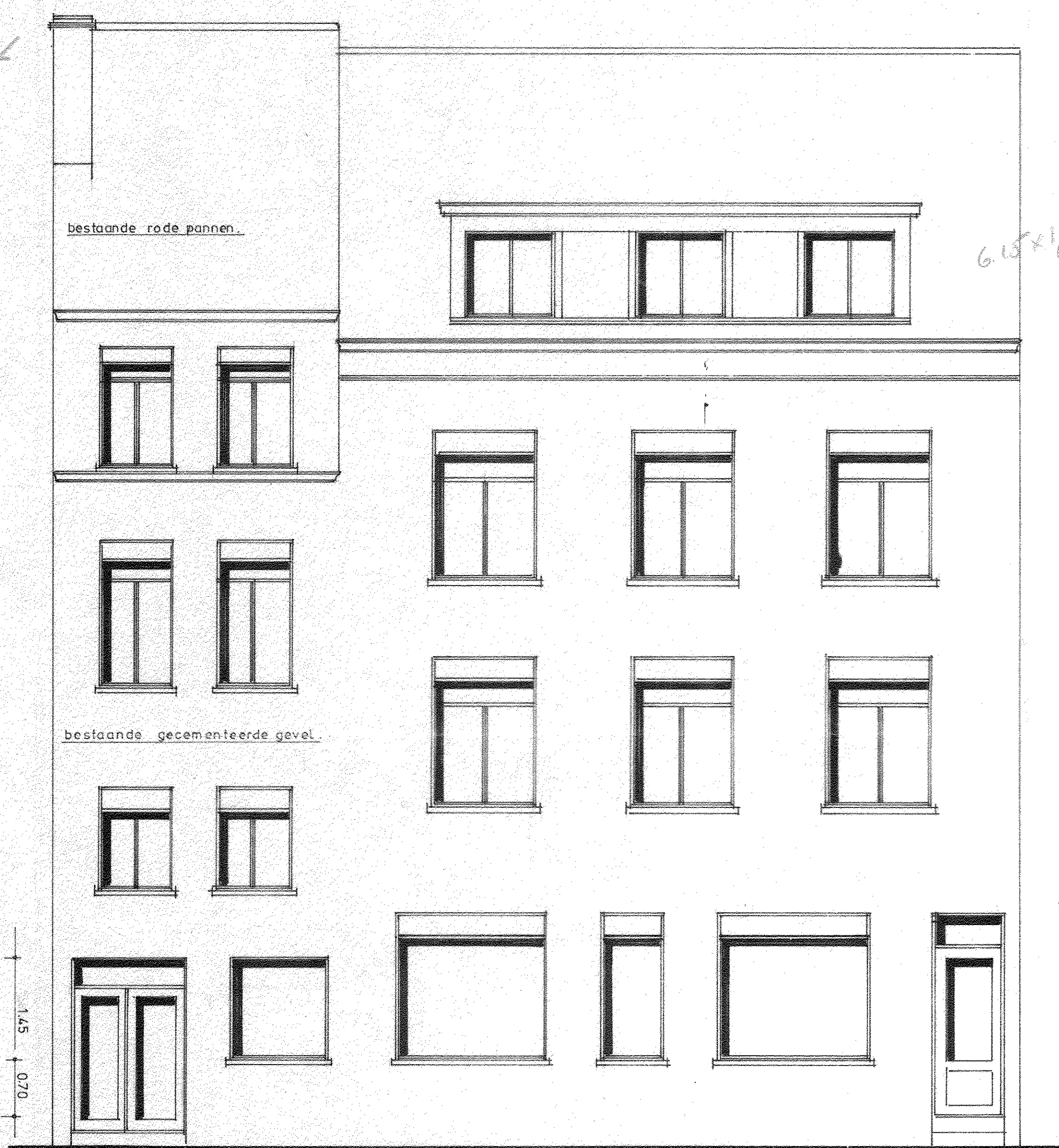
gewijzigde voorgevel.
