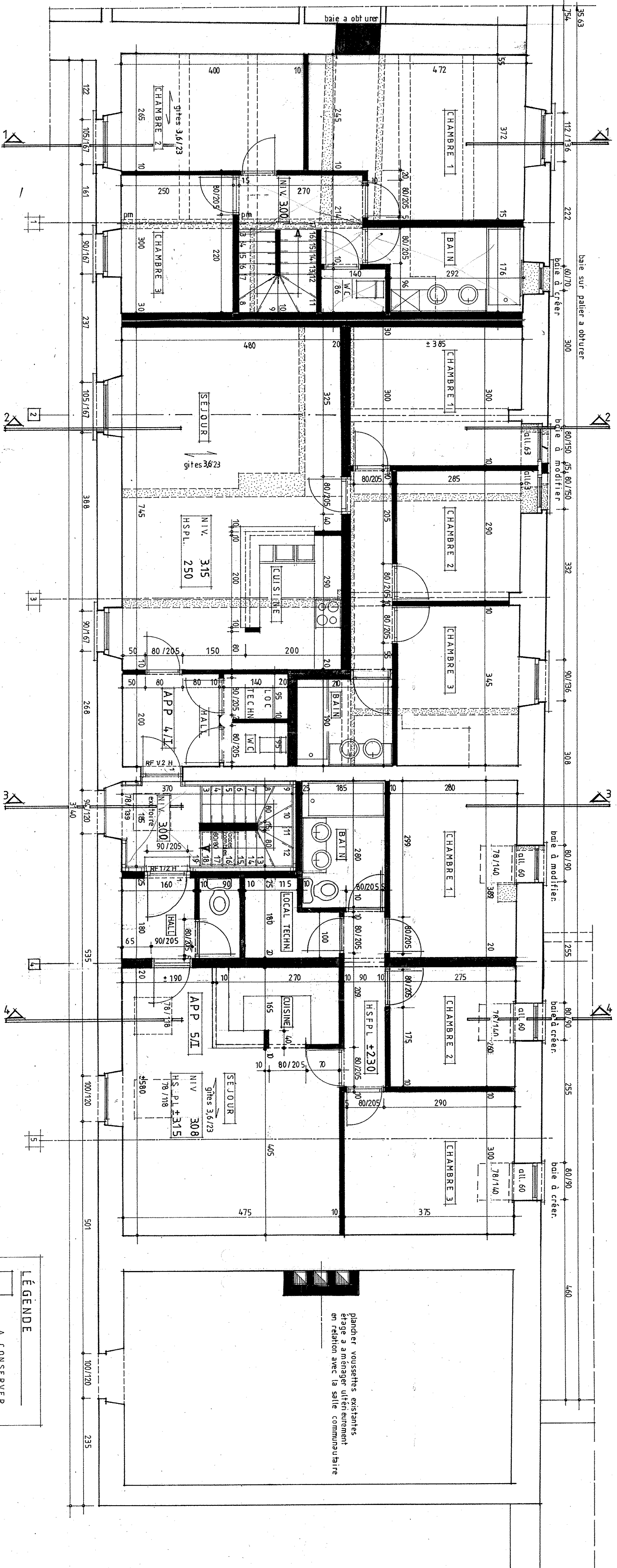
BATIMENT I. PLAN DE L'ETAGE.
