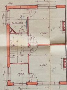
-VERDIEPING-
