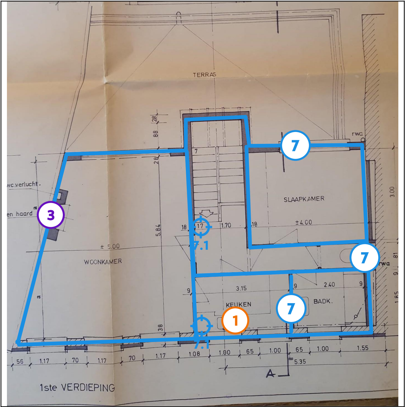
Legende van plan 1.1: eerste verdieping (muren)
