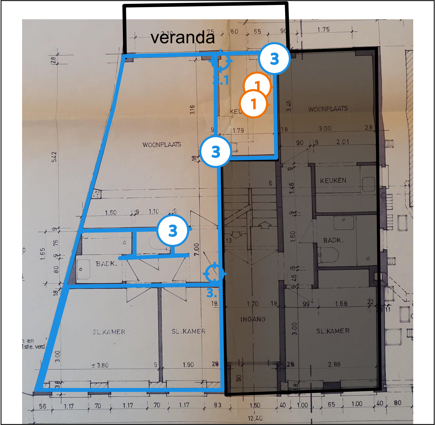
Legende van plan 1.1: gelijkvloers (muren)
