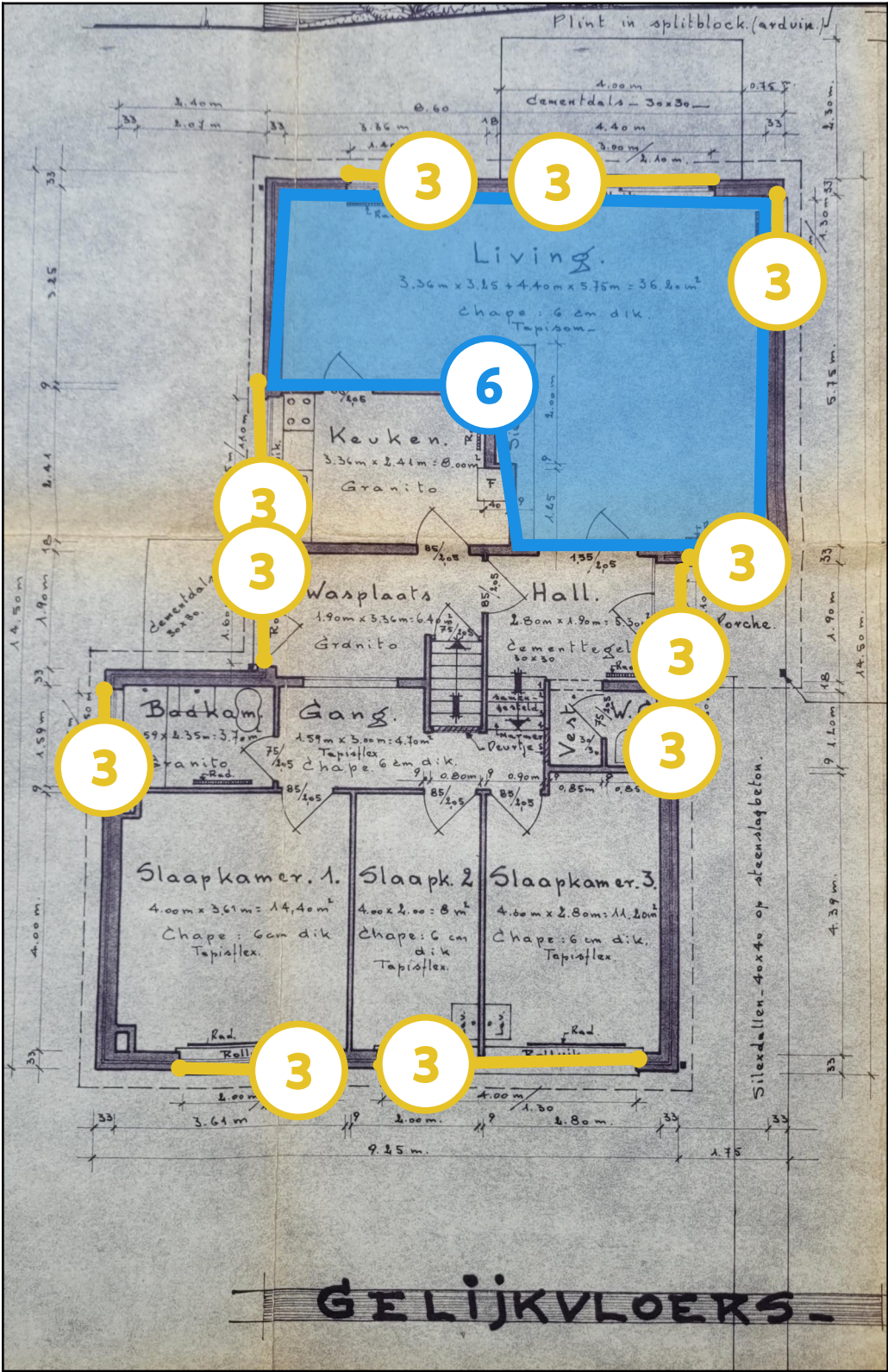
Legende van plan 1.3: gelijkvloers (vloer)
