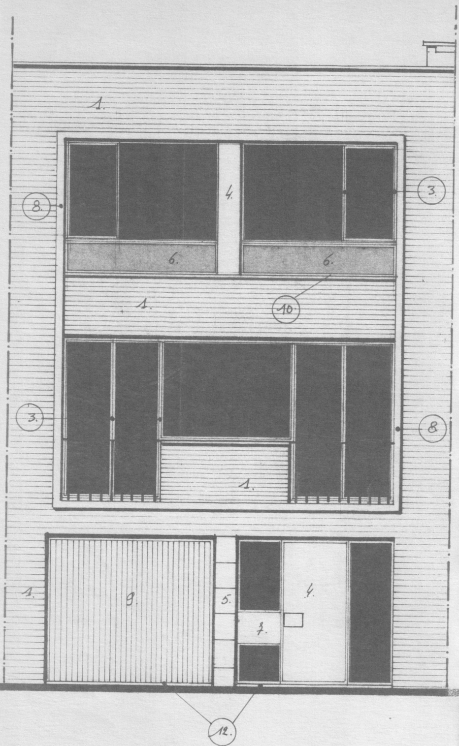
NOORD GEVEL.
