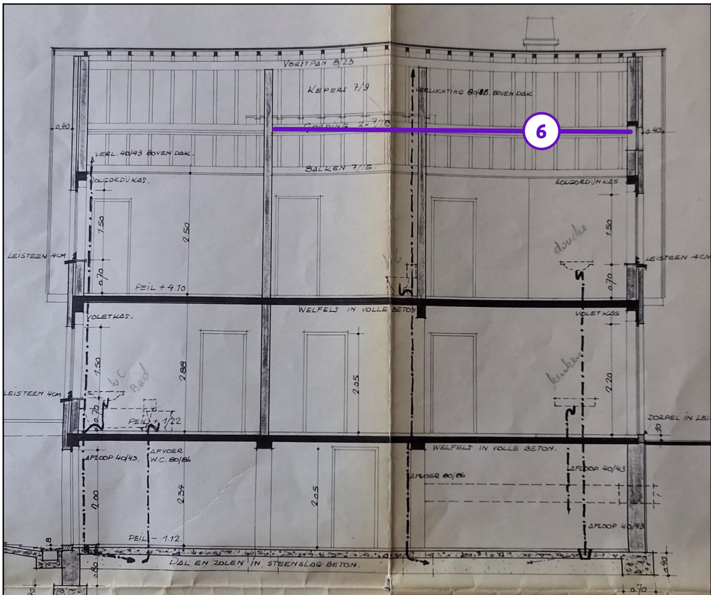
Legende van plan 1.9: Doorsnede
